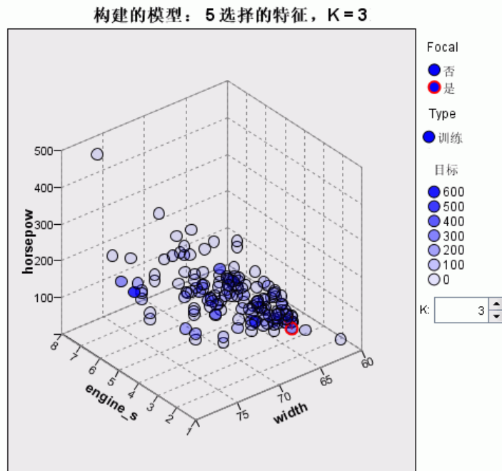
图片 16-10 预测变量空间
