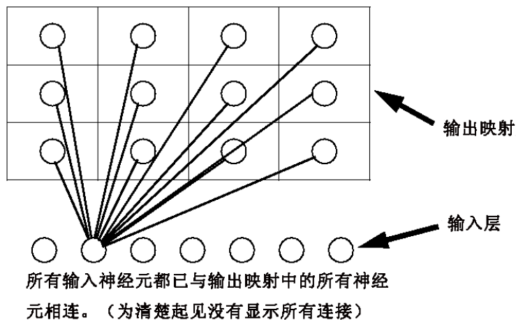
图片 11-2 Kohonen 网络的结构
