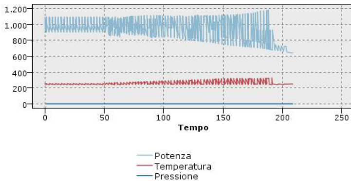
Figura 32. Multiplot standard che mostra la fluttuazione di una centrale elettrica nel tempo (si noti che senza la normalizzazione è impossibile vedere il grafico relativo alla pressione)
