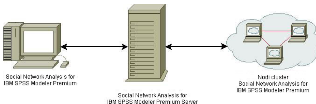
Figura 1. Architettura del prodotto
