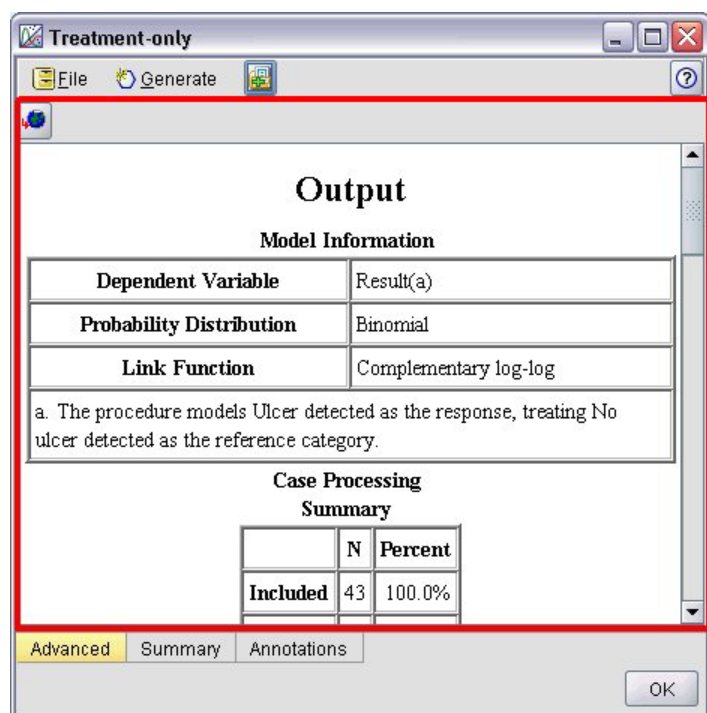
図 42. テキスト・ブラウザ・パネルが強調表示されたモデル出力ウィンドウ
