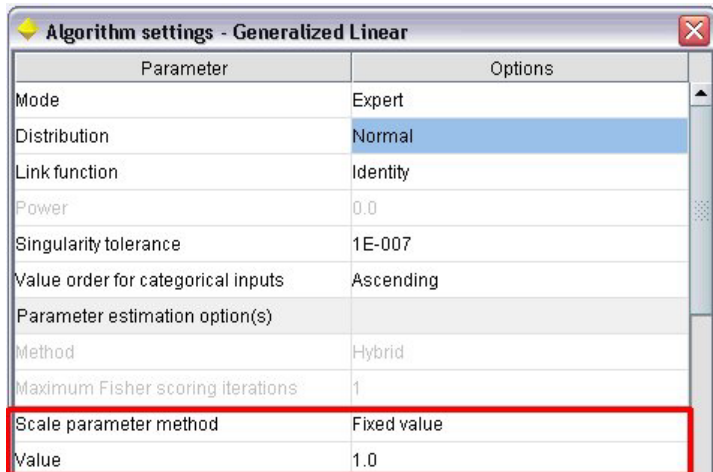
図 35. constraint の効果 - 有効化されたパラメーター
