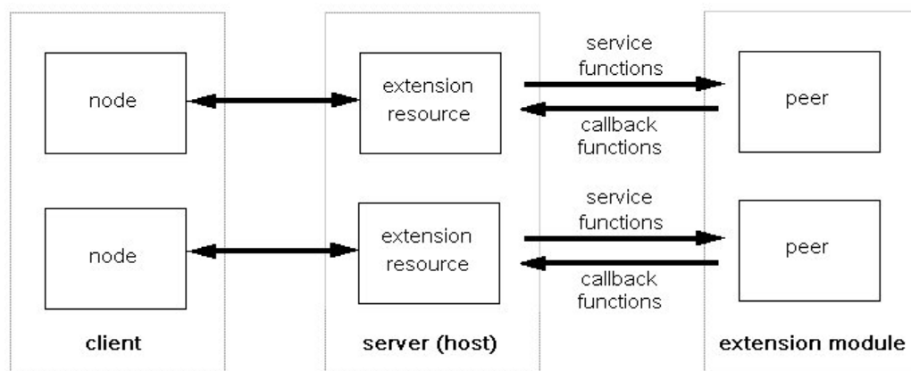
図 95. CLEF API アーキテクチャー
