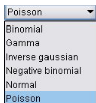
図 55. 選択情報
