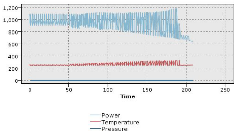
図 32. 時間の経過による発電装置の変動を示す標準の線グラフ (正規化を行わないと、圧力の作図は参照できないことに注意してください)
