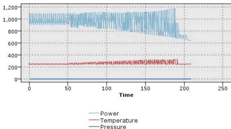
Рисунок 32. Стандартный график нескольких зависимостей, показывающий неравномерность работы силовой установки по времени (без нормализации; график для давления невиден)
