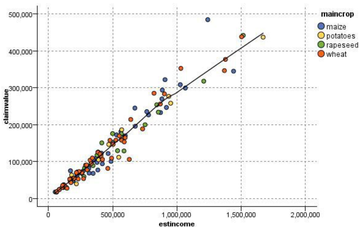
Рисунок 24. График с наложением сглаживателя LOESS
