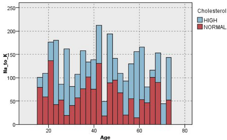
Рисунок 31. Диаграмма собрания, выводимая без оси z, но с выделенным цветом уровнем холестерина
