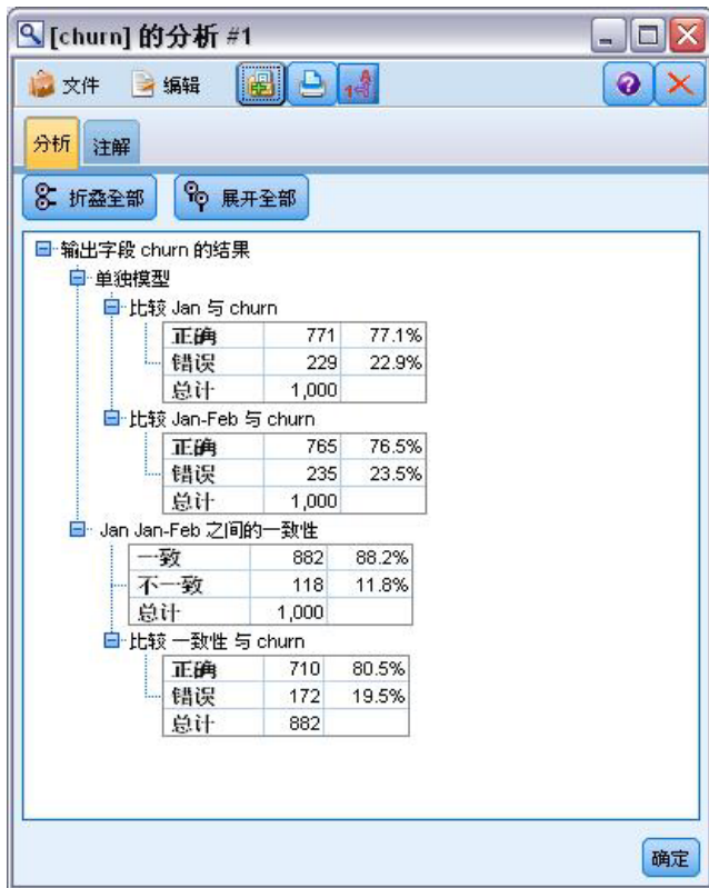
图 256. 分析模型准确性
