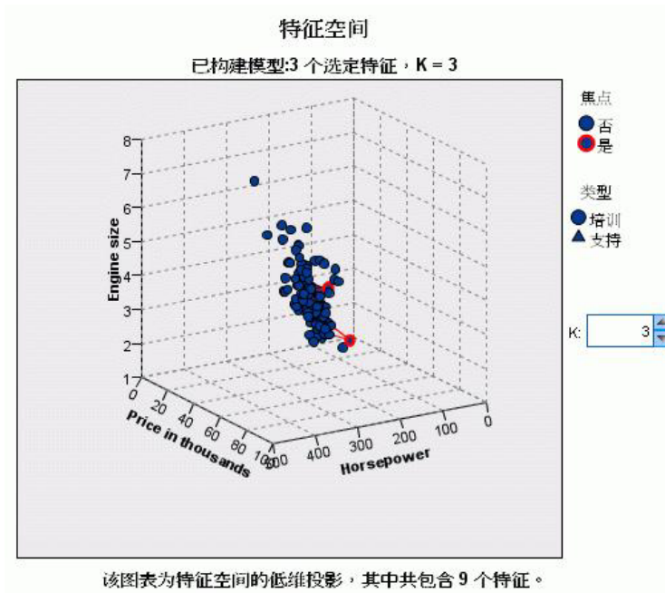
图 396. 预测变量空间图表
