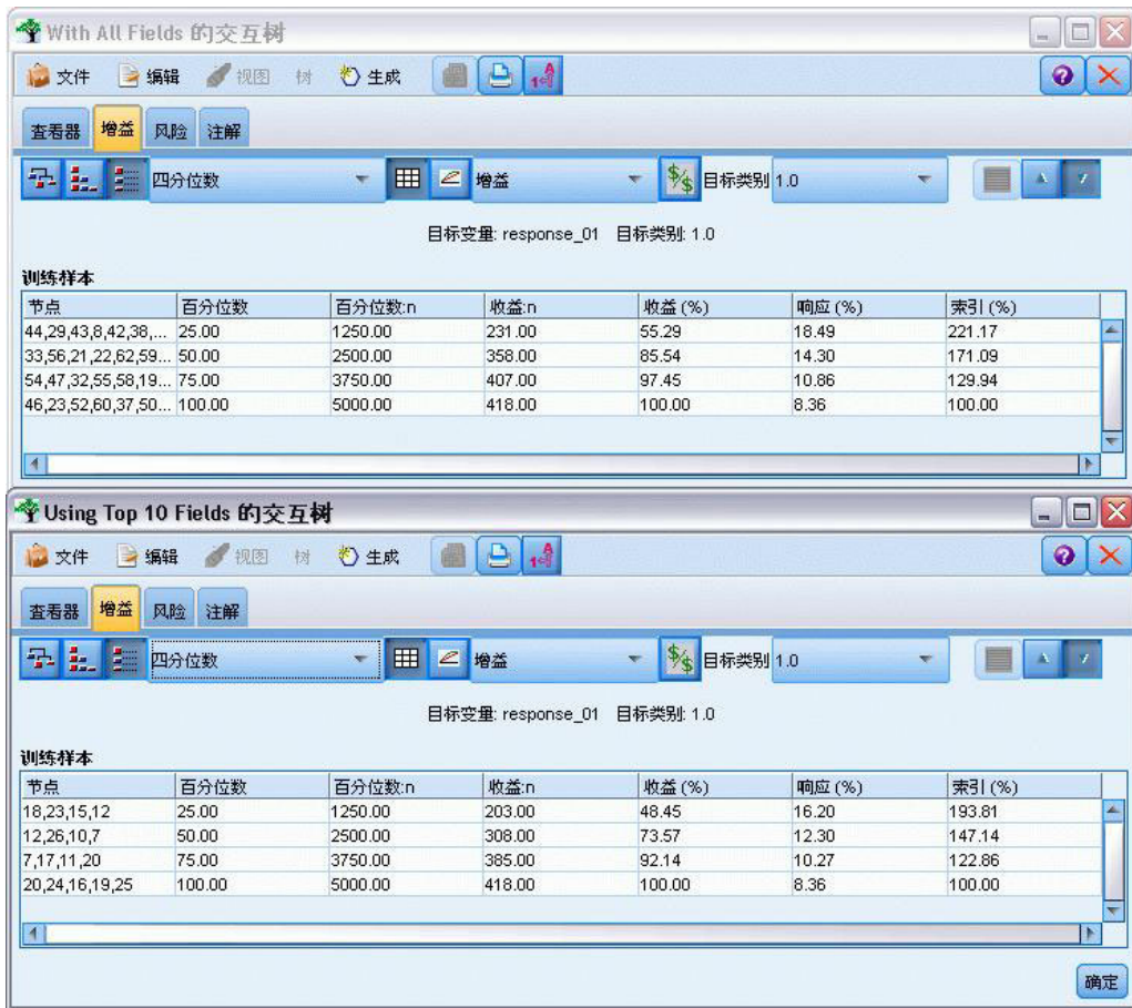
图 107. 两个 CHAID 模型的增益图
