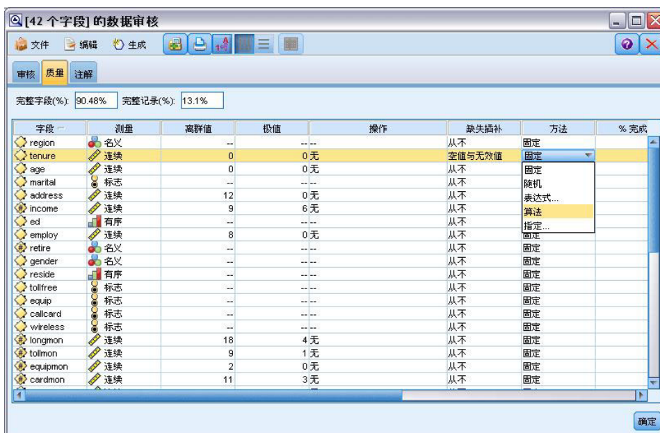
图 70. 选择插补方法
