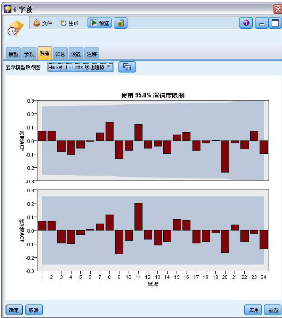
图 186. 市场的 ACF 值和 PACF 值
