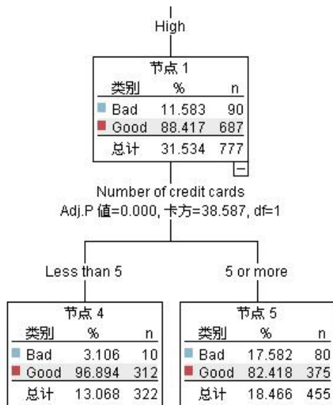
图 22. 高收入客户的树形视图
