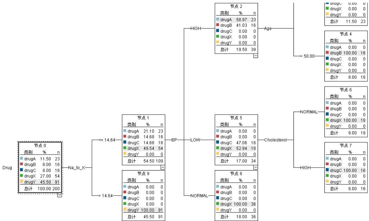
图 99. 图形形式的决策树
