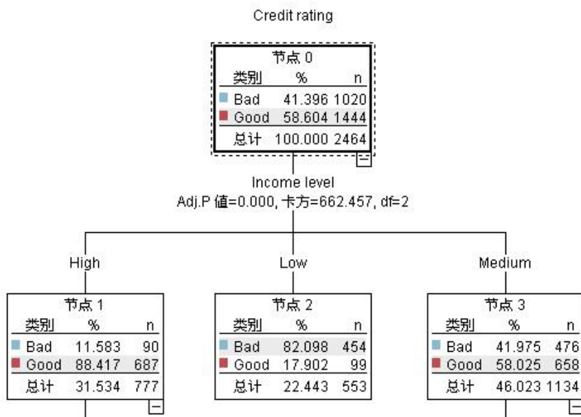
图 11. 简单的决策树模型
