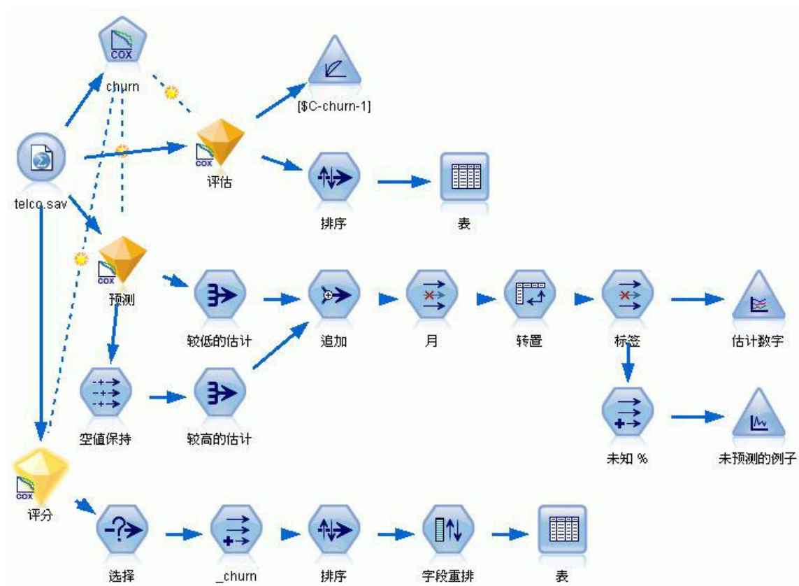
图 343. 用于分析流失时间的样本流
