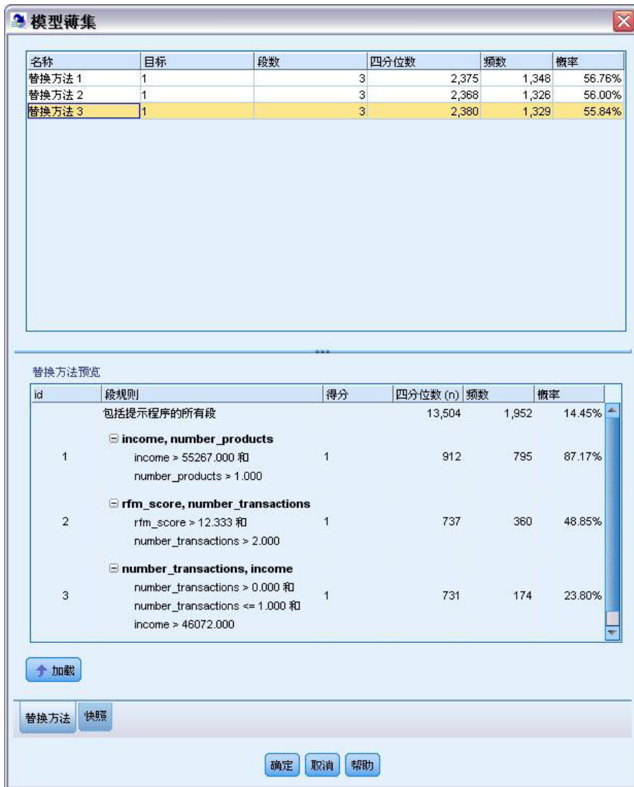
图 124. 可用替代模型
