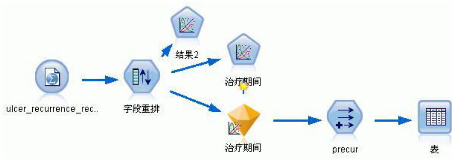
图 299. 用于预测溃疡复发的样本流
