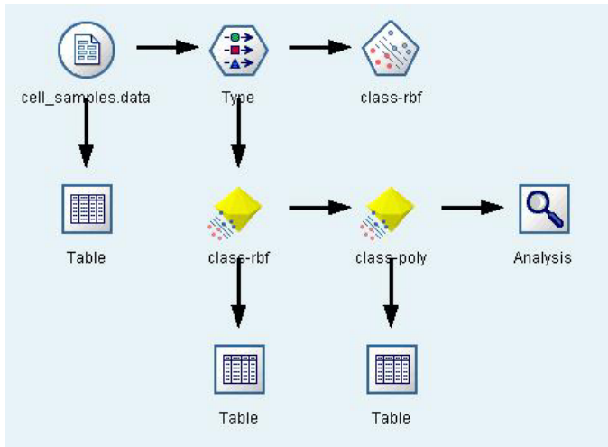
图 331. 用于显示 SVM 建模的样本流
