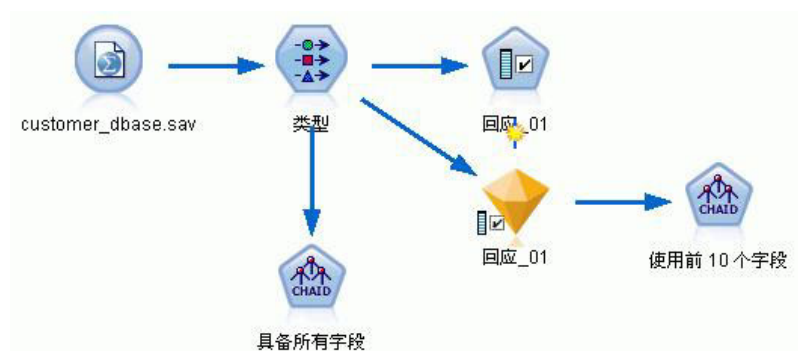
图 102. “特征选择”示例流
