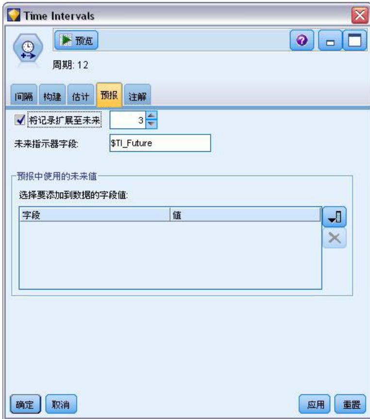
图 193. 检查预测期的设置
