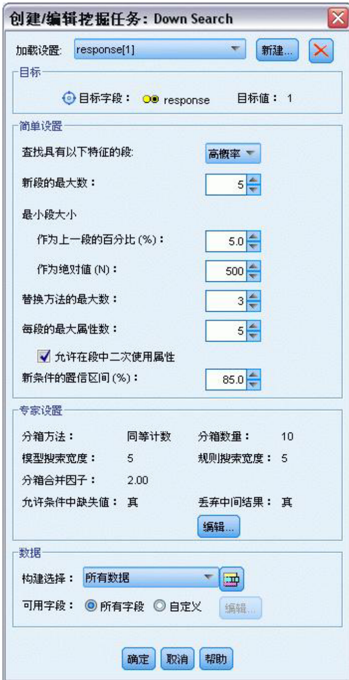
图 132. 选择缺省挖掘任务
