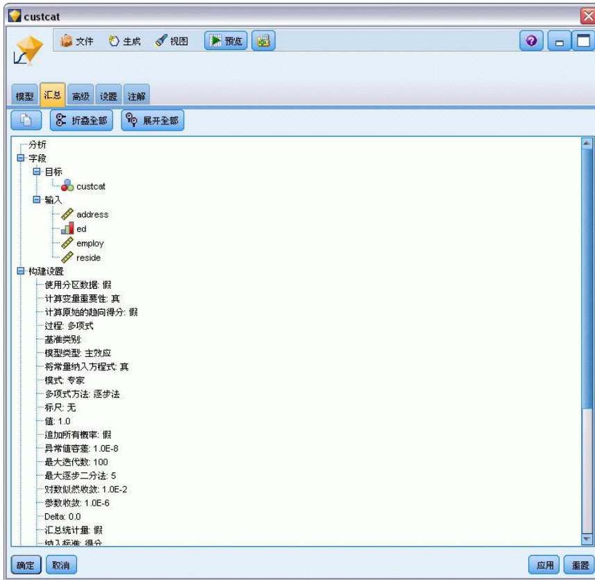
图 151. 显示目标字段和输入字段的模型摘要
