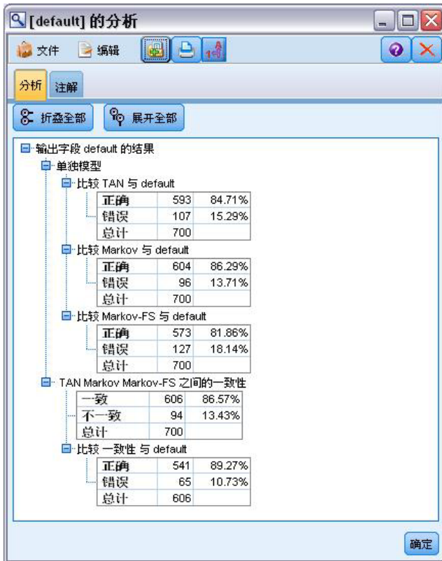
图 243. 分析模型准确性
