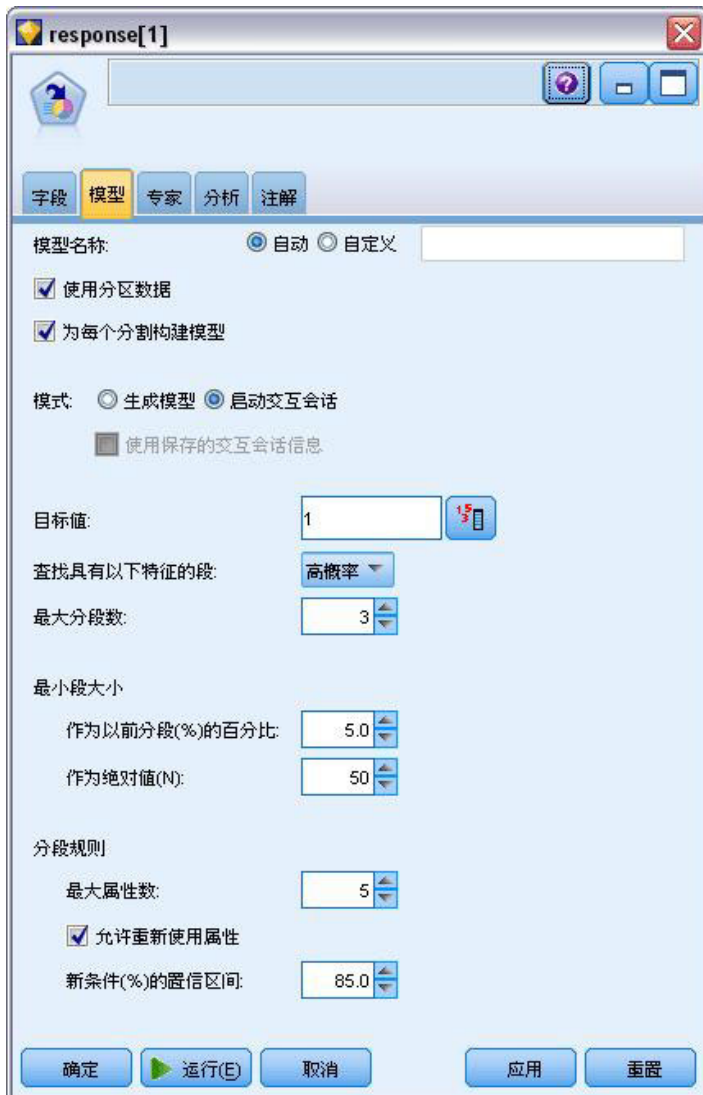
图 120. “决策列表”节点，“模型”选项卡
