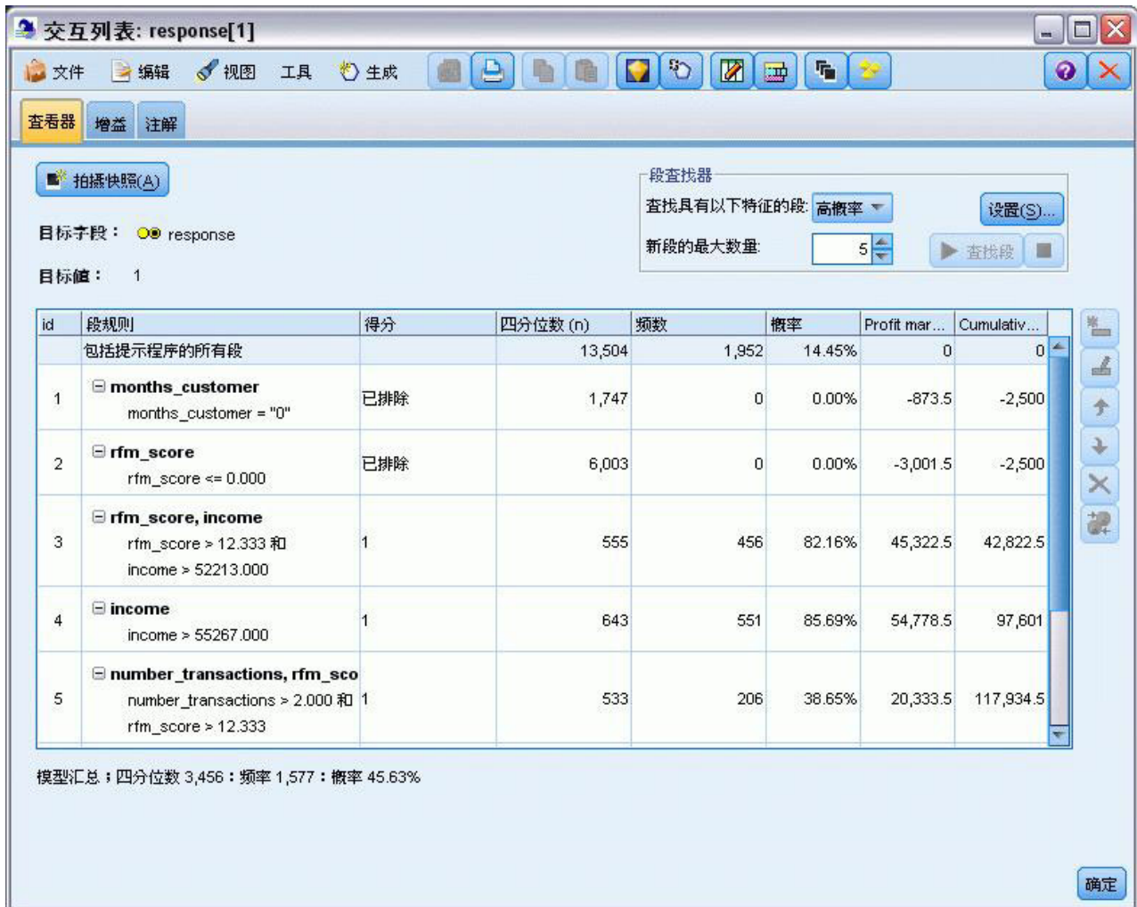
图 140. “交互列表”查看器中显示的 Excel 定制测量
