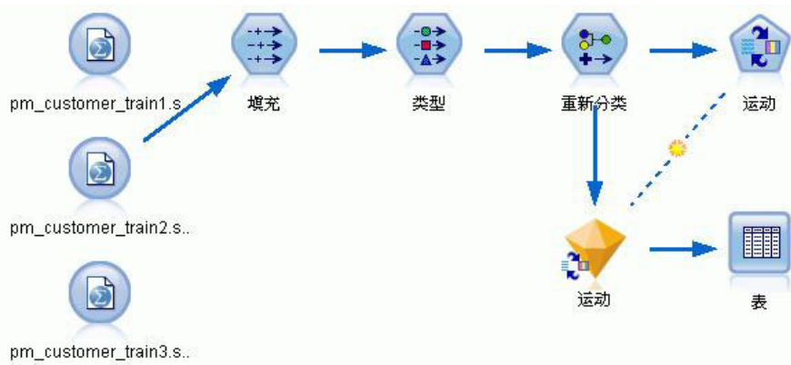
图 228. 将第二个数据源附加到 SLRM 流
