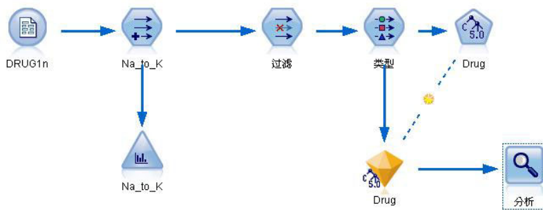
图 100. 添加“分析”节点
