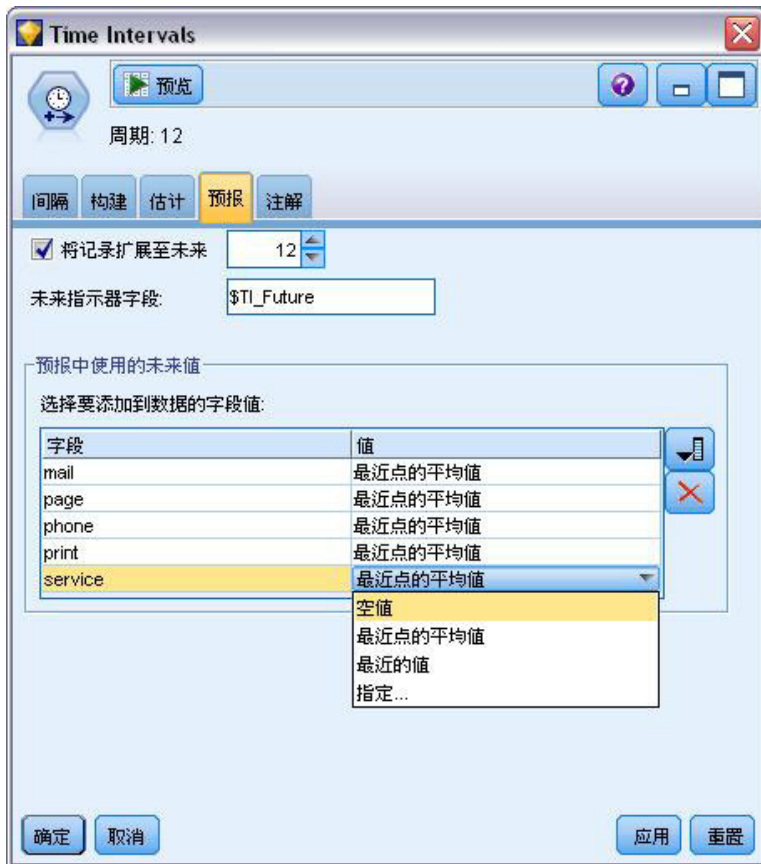
图 218. 指定预测变量字段的未来值
