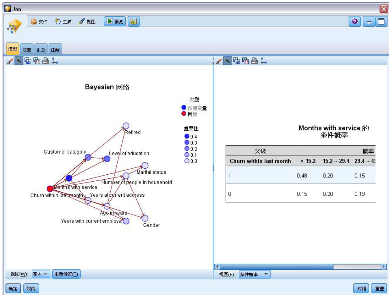
图 254. 显示条件概率的贝叶斯网络模型
