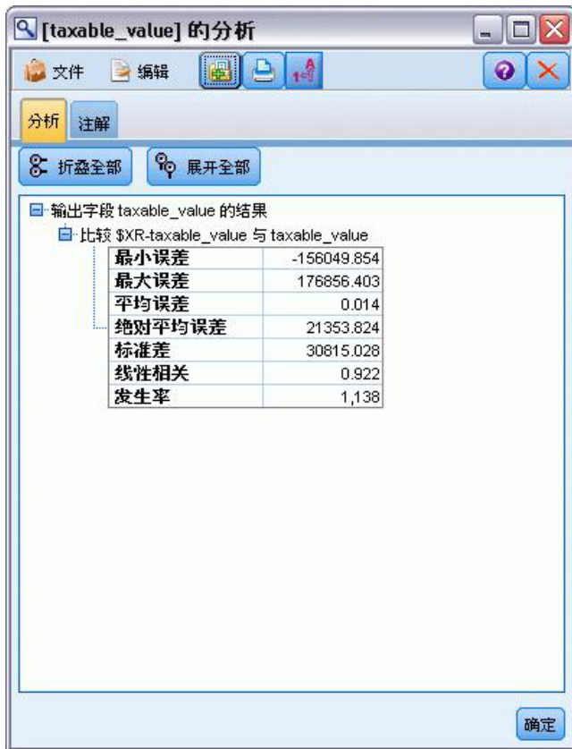
图 49. 自动数值样本流
