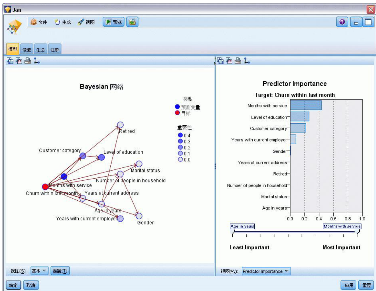
图 253. 显示预测变量重要性的贝叶斯网络模型
