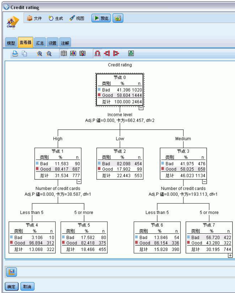
图 21. 模型块中的查看器选项卡，已选择缩小
