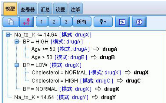
图 98. 完全展开的规则浏览器
