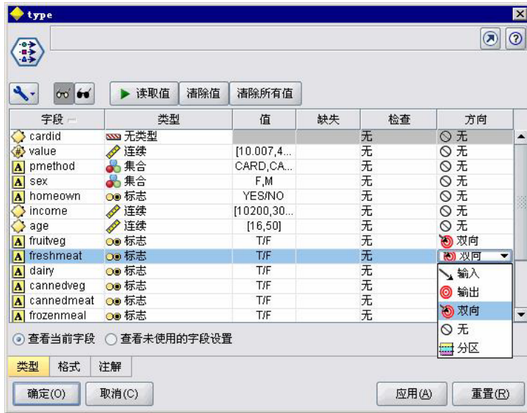
图 385. 选择用于建模的字段
