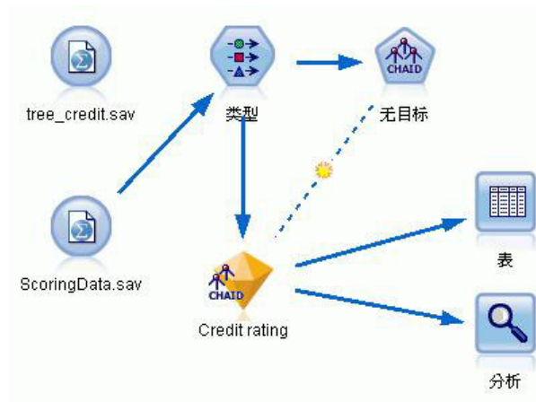
图 28. 附加用于评分的新数据
