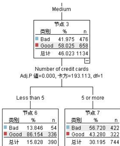
图 23. 中等收入客户的树形视图
