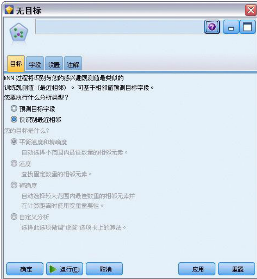
图 393. 选择识别最近相邻元素
