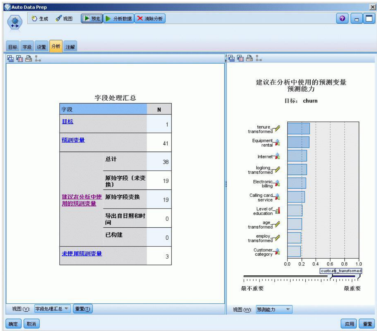
图 54. 数据处理摘要
