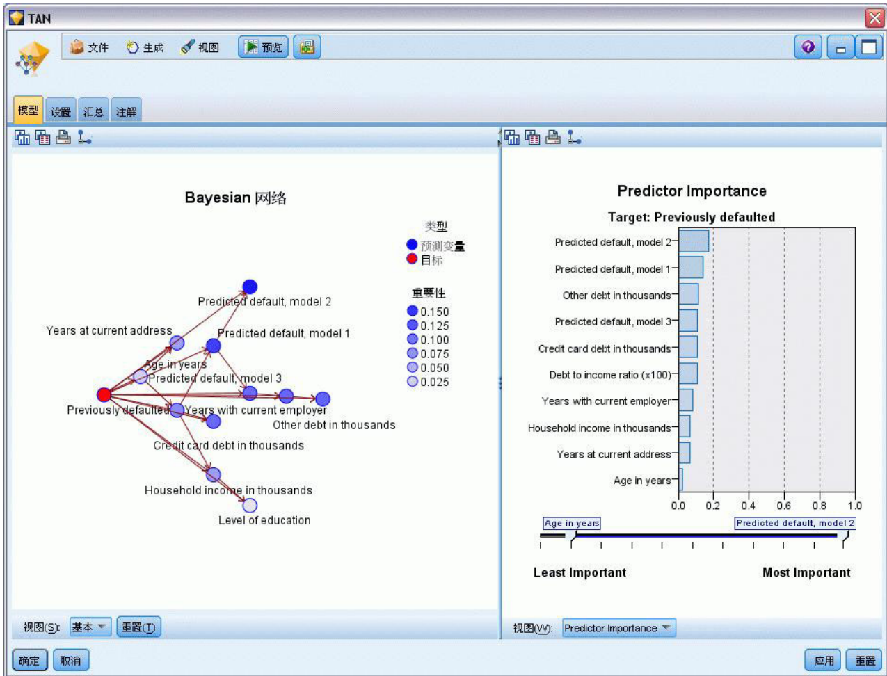
图 239. 查看树扩展朴素贝叶斯模型
