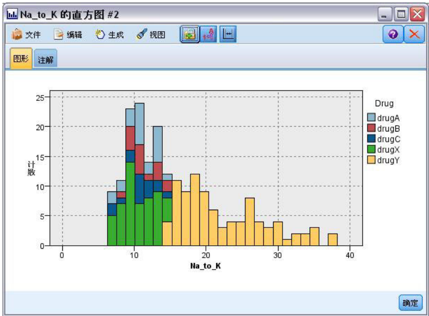
图 2. 示例直方图
