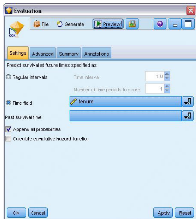
Figure 357. Nugget de Cox : Onglet Paramètres
