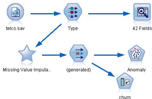
Figure 76. Flux avec super noeud Valeurs manquantes
