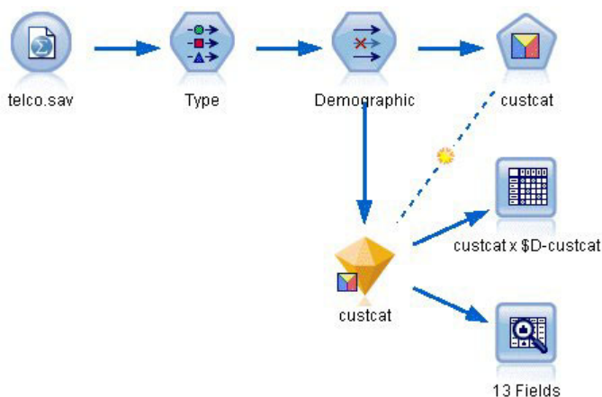
Figure 269. Flux d'échantillons permettant de classier les clients par analyse discriminante
