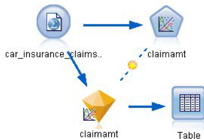
Figure 326. Flux d'échantillons relatif à la prévision des déclarations de sinistre automobile
