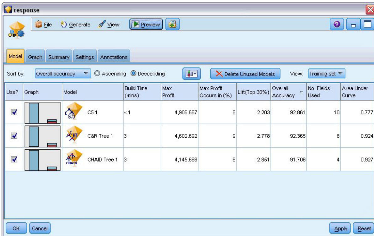
Figure 40. Résultats du Discriminant automatique
