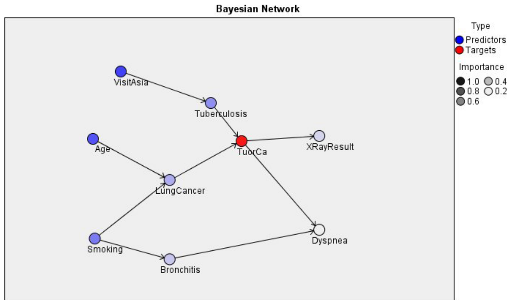
Figure 29. Exemple du réseau Asiatique de Lauritzen et Spiegelhalter
