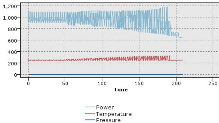
Figure 26. Graphique Courbes standard indiquant les variations de la centrale électrique dans le temps (sans normalisation, il est impossible de visualiser le tracé concernant la pression)
