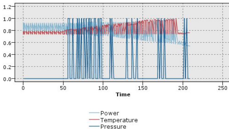
Figure 27. Graphique Courbes normalisé montrant le tracé de la pression
