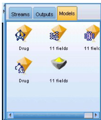
Рисунок 26. Палитра моделей
