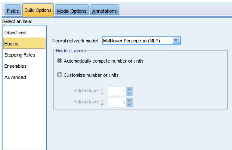
Рисунок 33. Основные параметры
