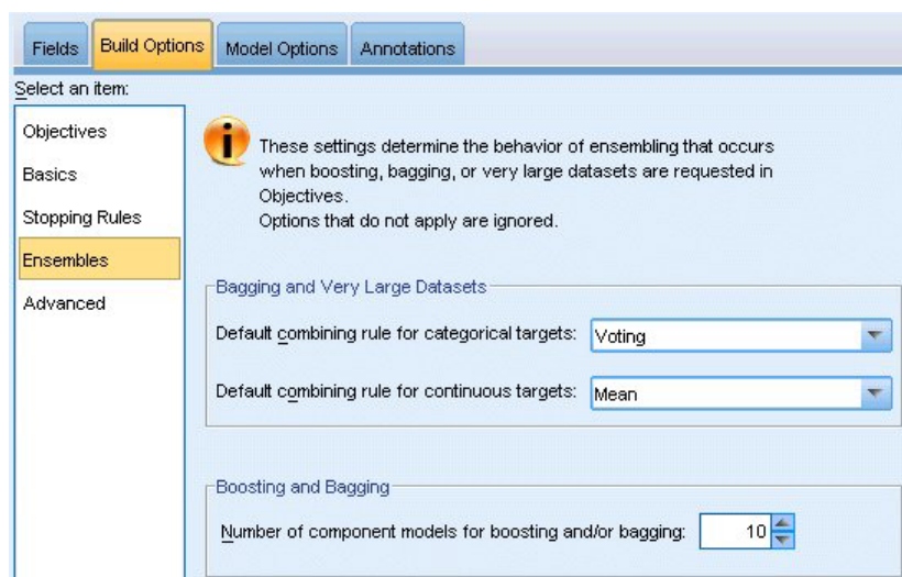
Рисунок 35. Параметры ансамблей
