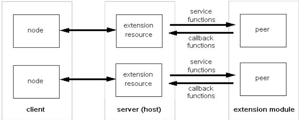
Abbildung 95. CLEF API-Architektur
