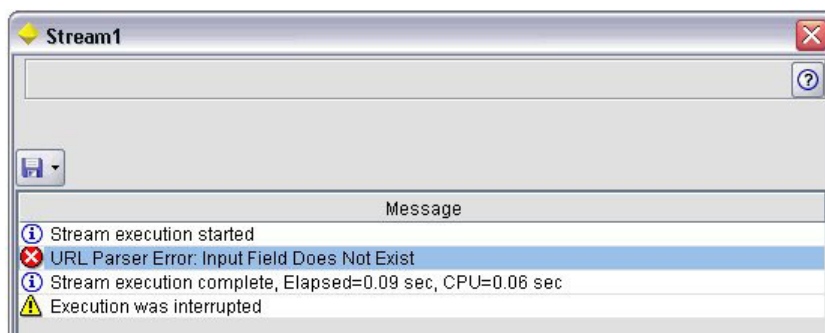
Abbildung 29. Fehlermeldungsanzeige
