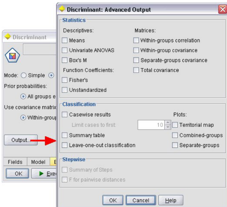
Abbildung 50. Eigenschaftsunterfenster
