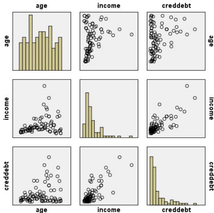
図 17. 散布図行列 (SPLOM)
