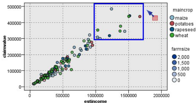
図 57. 申請値の高い領域の定義
