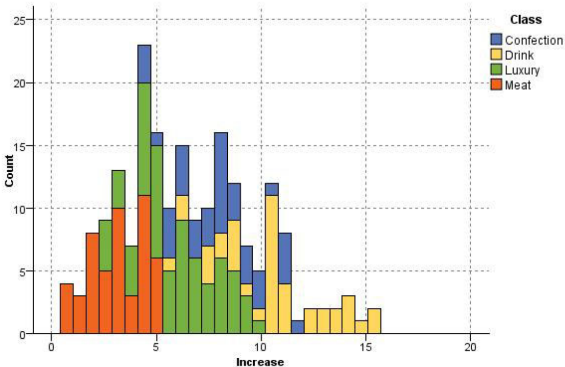
図 33. プロモーションによる購入の増加の分布をカテゴリー別に表したヒストグラム
