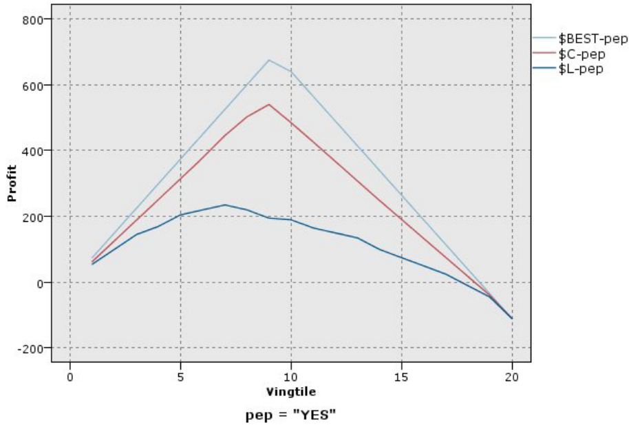
図 46. ベスト・ラインが表示された利益グラフ (累積)
