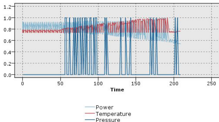
図 27. 圧力の作図を表示する正規化された線グラフ
