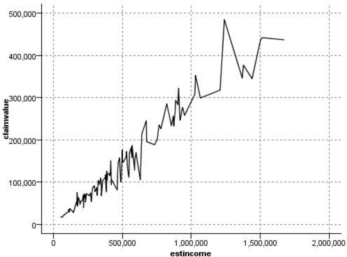
図21. 「X モード」を「ソート」に設定した折れ線
