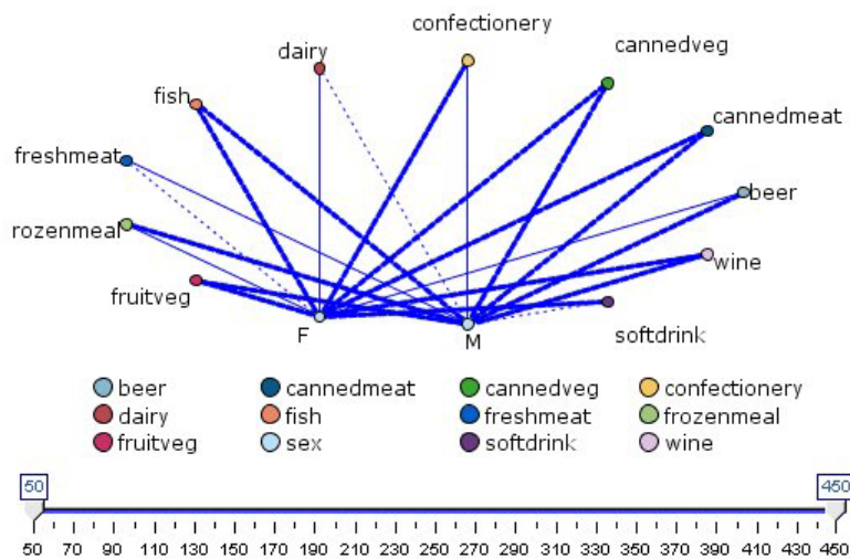
図 38. 購入された食料雑貨品と性別の関係を表した Web グラフ
