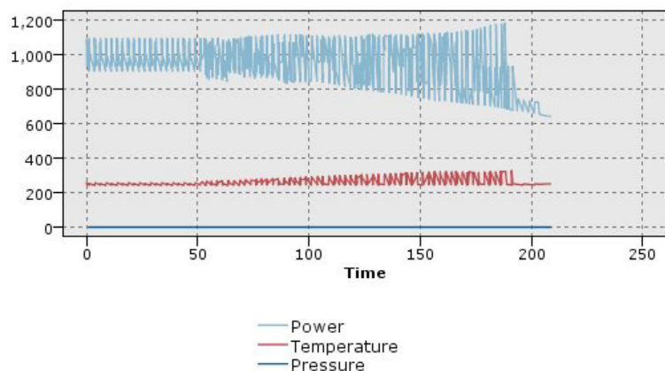
図 26. 時間の経過による発電装置の変動を示す標準の線グラフ (正規化を行わないと、圧力の作図は参照できないことに注意してください)
