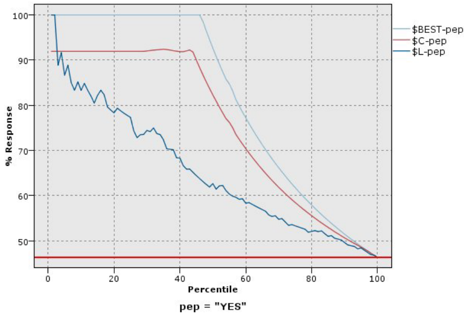
図 45. ベスト・ラインが表示された回答グラフ (累積)
