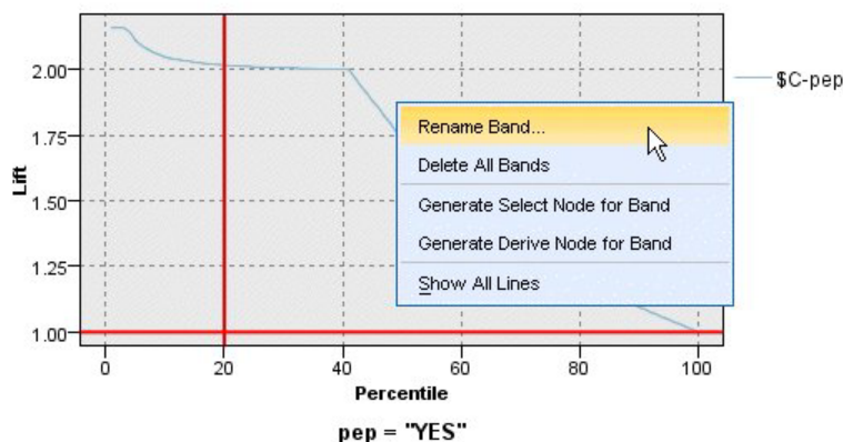
図 49. 評価グラフの作業
