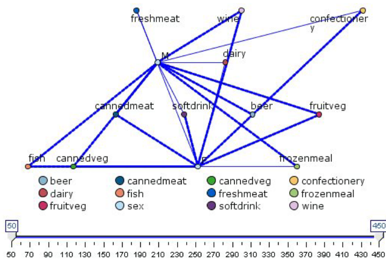
図 39. 冷凍食品と缶詰野菜から他の食料雑貨への強いリンクを表した Web グラフ
