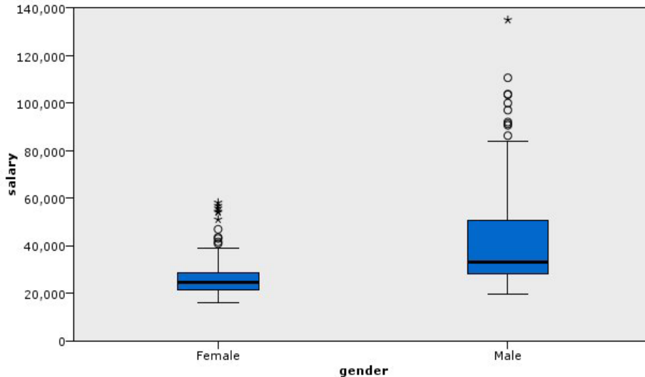
図 14. Boxplot
