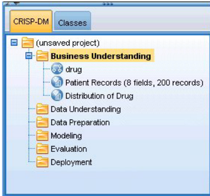
그림 8. CRISP-DM 보기
