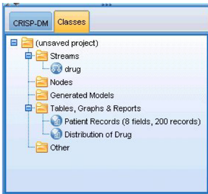
그림 9. 클래스 보기
