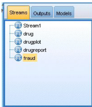
Рисунок 5. Вкладка Поток
