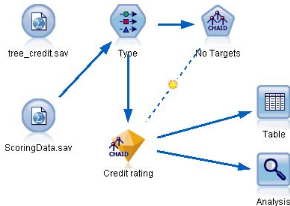
Figura 18. Anexando novos dados para escoragem
