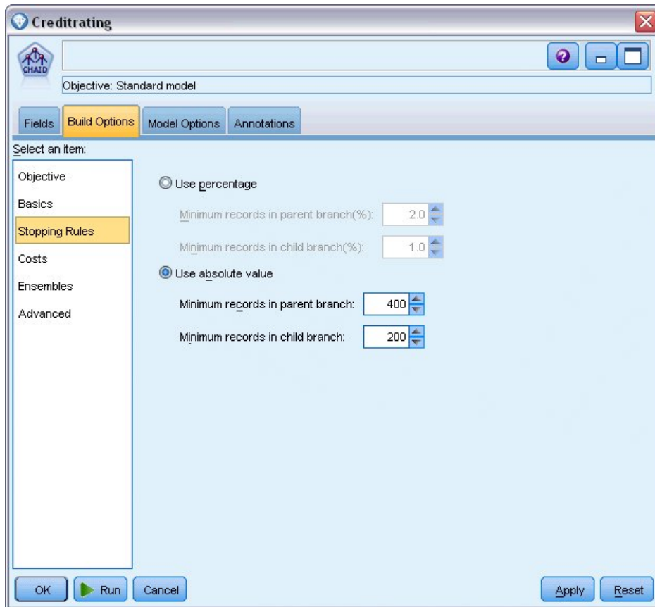
Figura 7. Configurando os critérios de parada para construção de árvore de decisão
