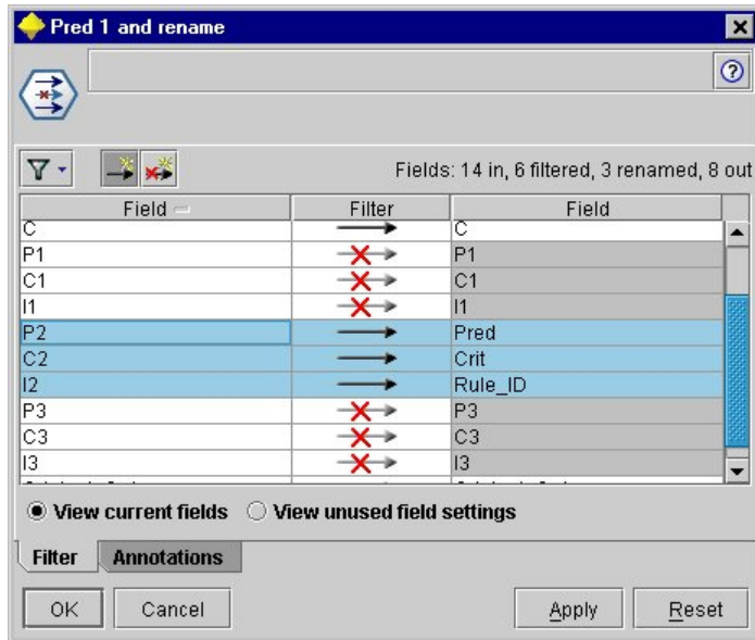
Figura 50. Filtrando campos para as previsões 1 e 3 enquanto renomeia campos para a previsão 2.
