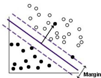
Abbildung 65. Problem bei linearer Trennung
