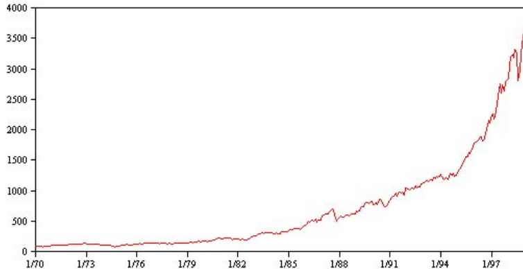
Abbildung 53. Trend
