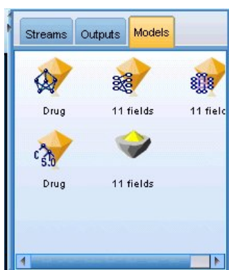
Abbildung 26. Modellpalette
