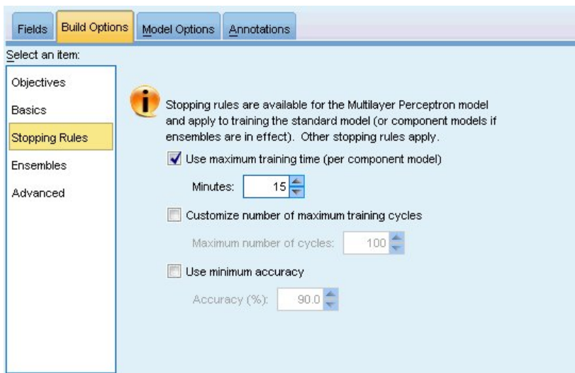
Abbildung 34. Stoppregeln - Einstellungen
