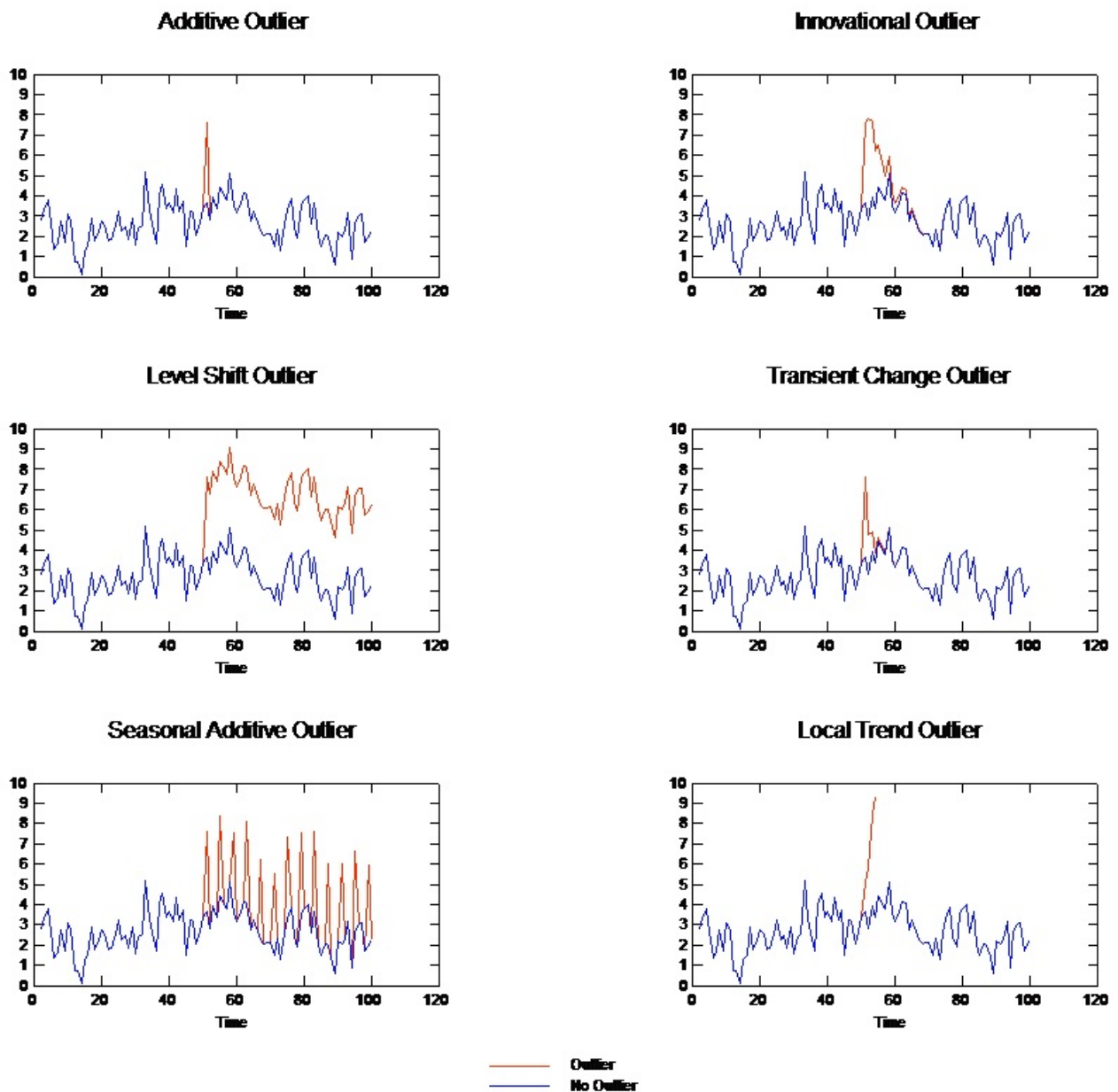
Abbildung 57. Ausreißertypen
