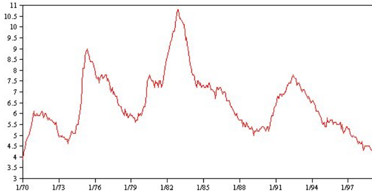
Figura 55. Ciclo no estacional
