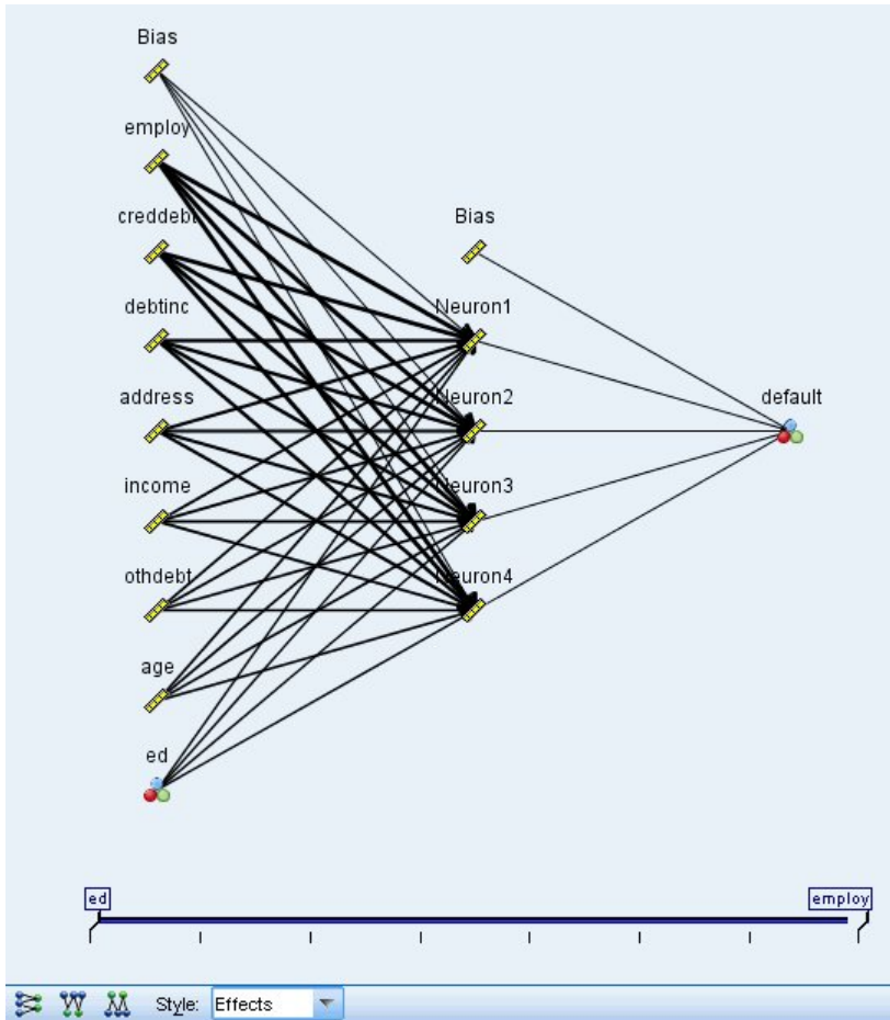
Figura 42. Visualizzazione Rete, input a sinistra, stile effetti
