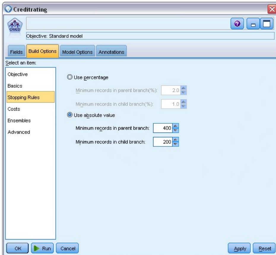
Figura 7. Impostazione dei criteri di arresto per la creazione di strutture ad albero delle decisioni
