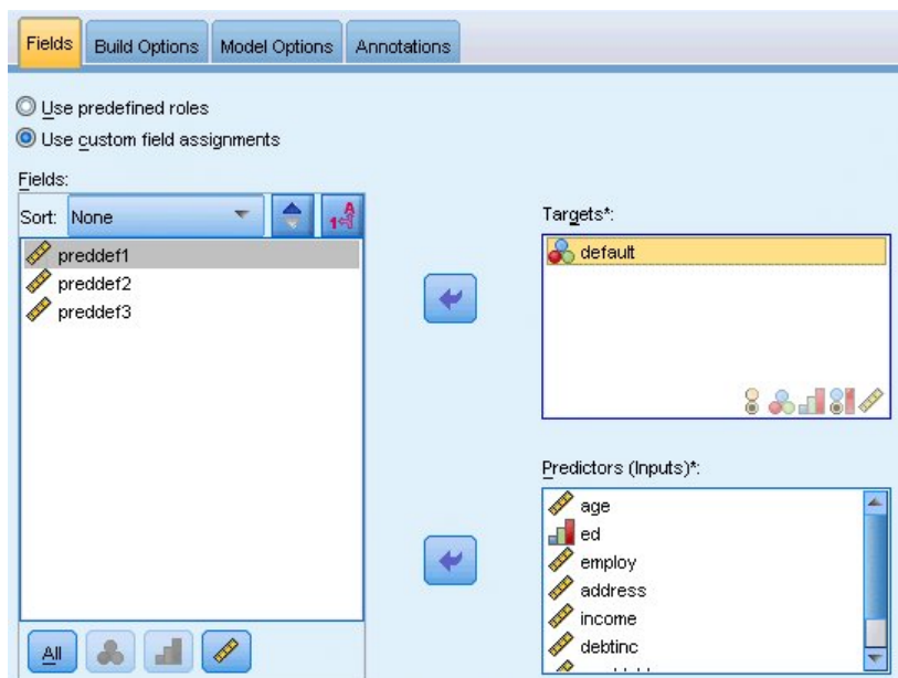
Figura 30. Scheda Campi
