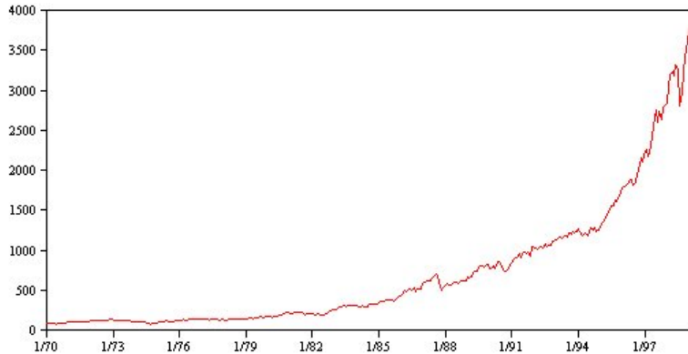
Figura 53. Tendenza
