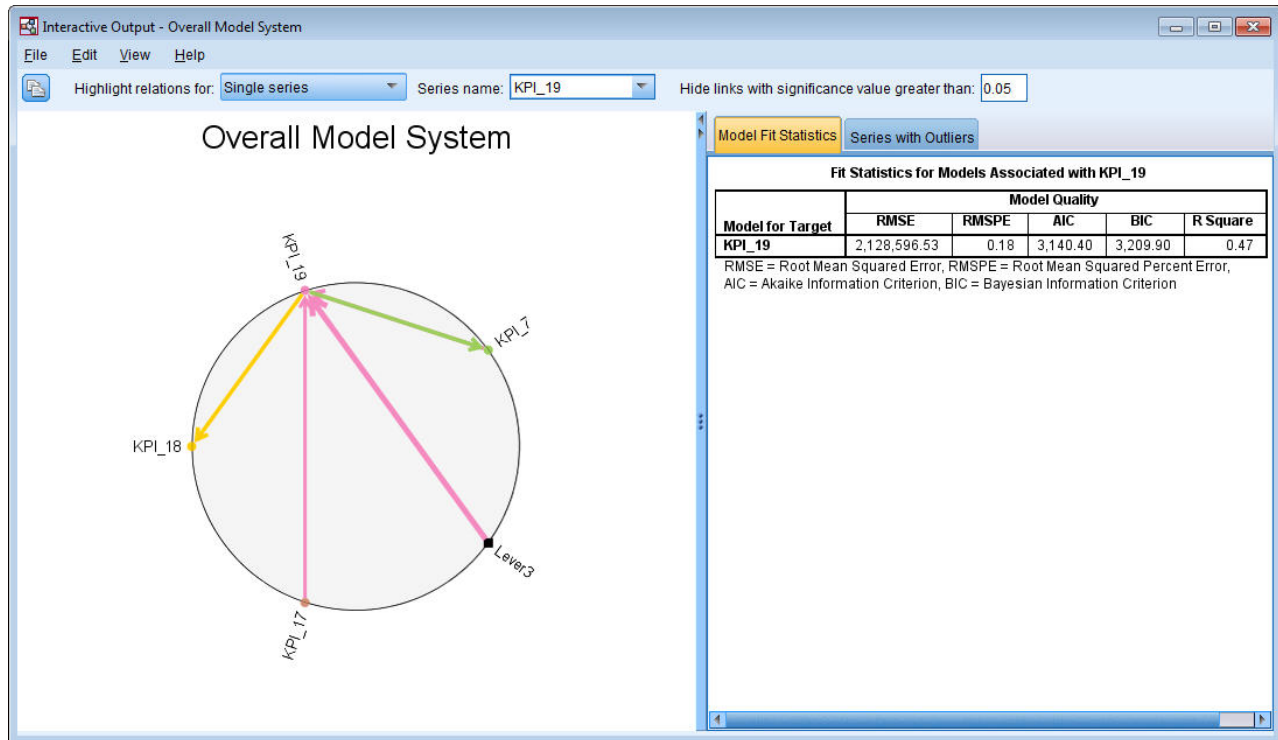
図 406. 全体のモデル システム、単一系列の表示
