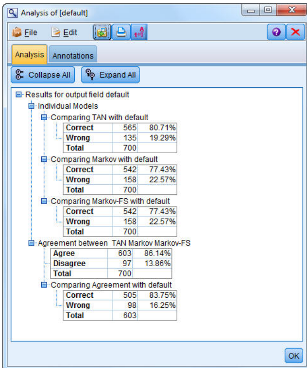
図 243. モデルの精度分析
