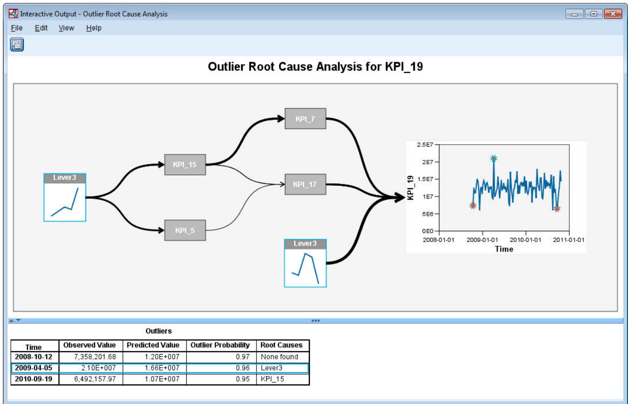
図 412. KPI_19 の外れ値の根本原因分析
