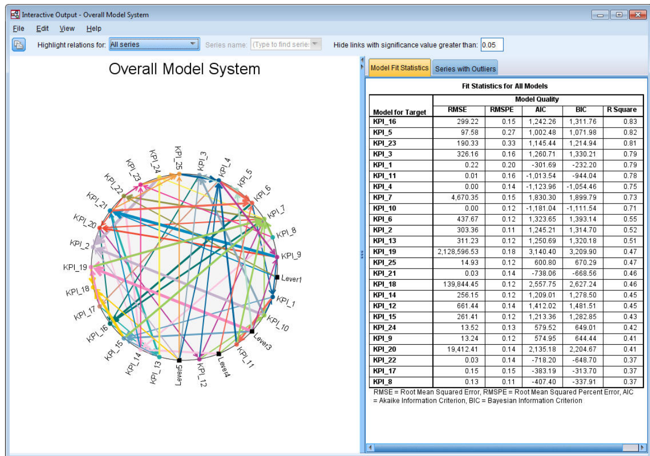
図 405. 全体のモデル システム、すべての系列の表示
