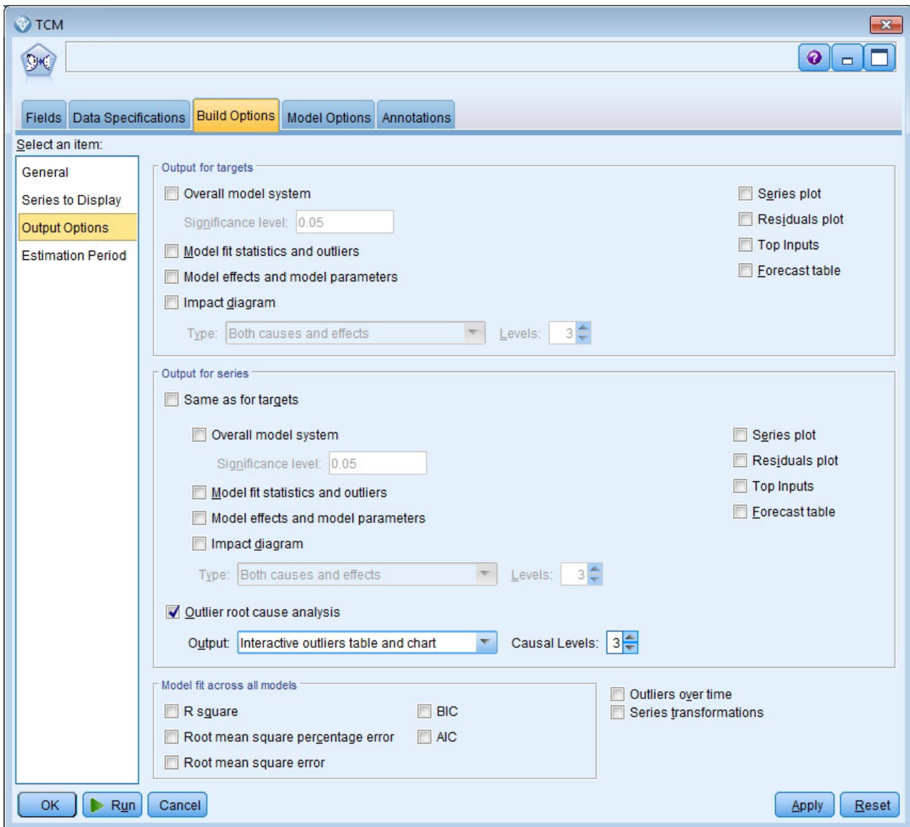
図 411. 時間的因果モデルの出力オプション
