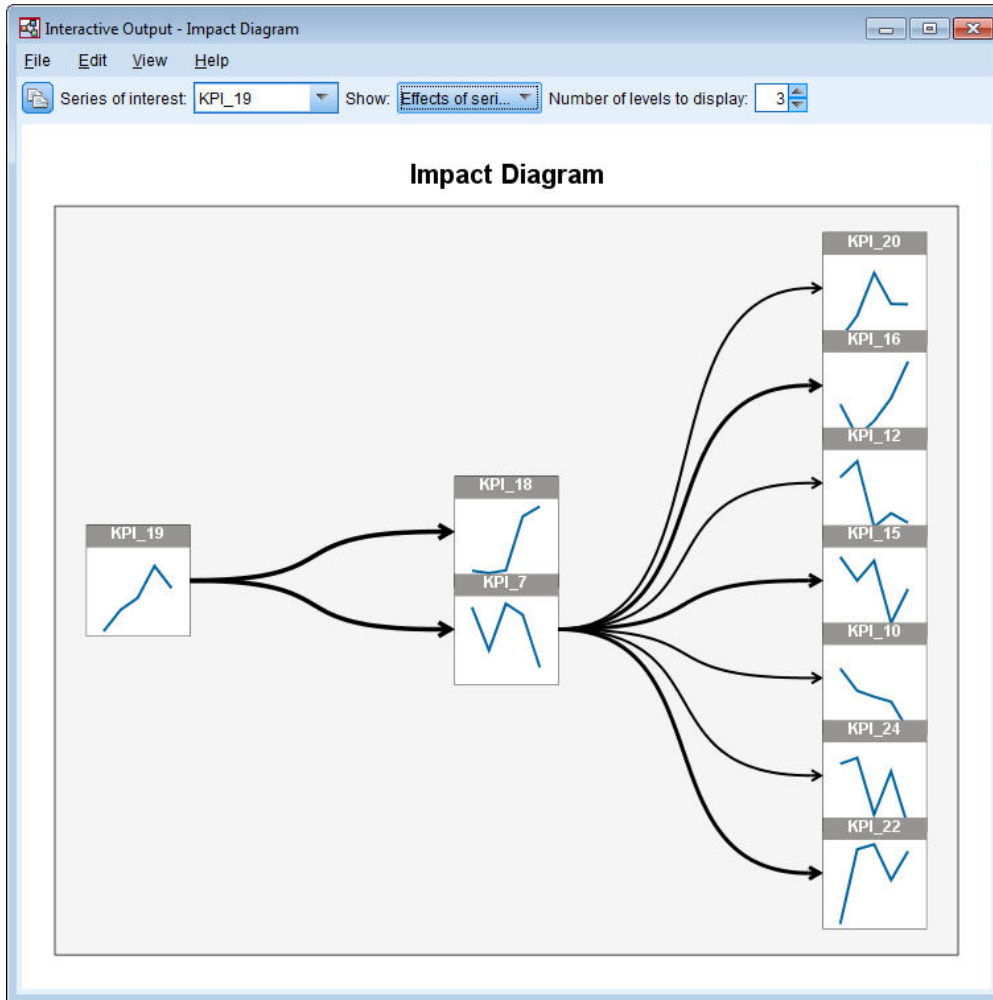
図 408. 効果の影響図
