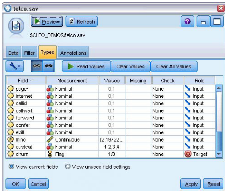
図 345. フィールドの役割の設定
