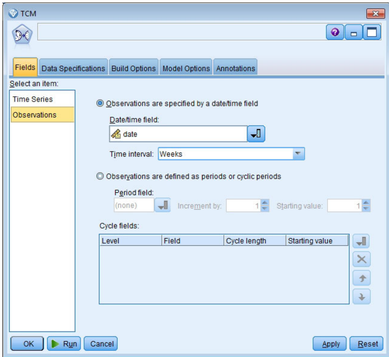
図 403. 時間的因果モデリング、観測
