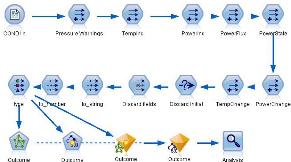
図 267. 学習済みのネットワークのテスト
