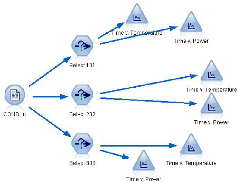
図 263. Condplot ストリーム
