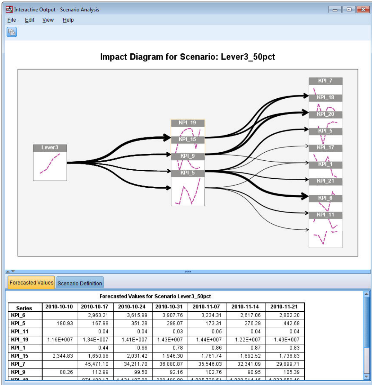
図 416. シナリオ: Lever3_50pct の影響図
