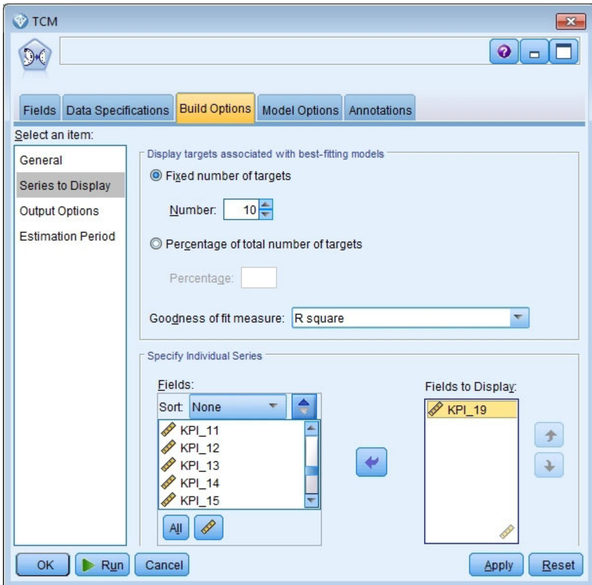
図 410. 時間的因果モデルの表示する系列
