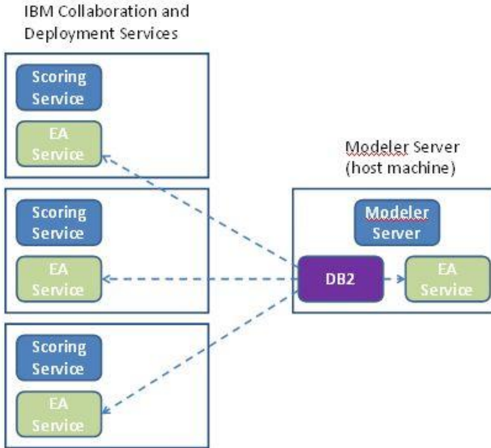
그림 1 - C&DS - 군집 시스템의 구성
