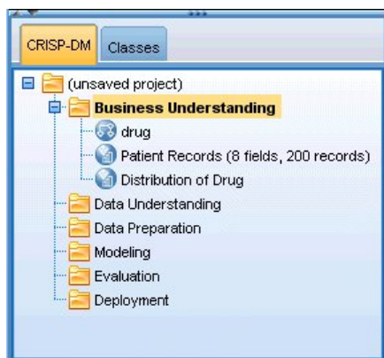
Рисунок 8. Представление CRISP-DM
