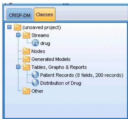
Рисунок 9. Представление классов
