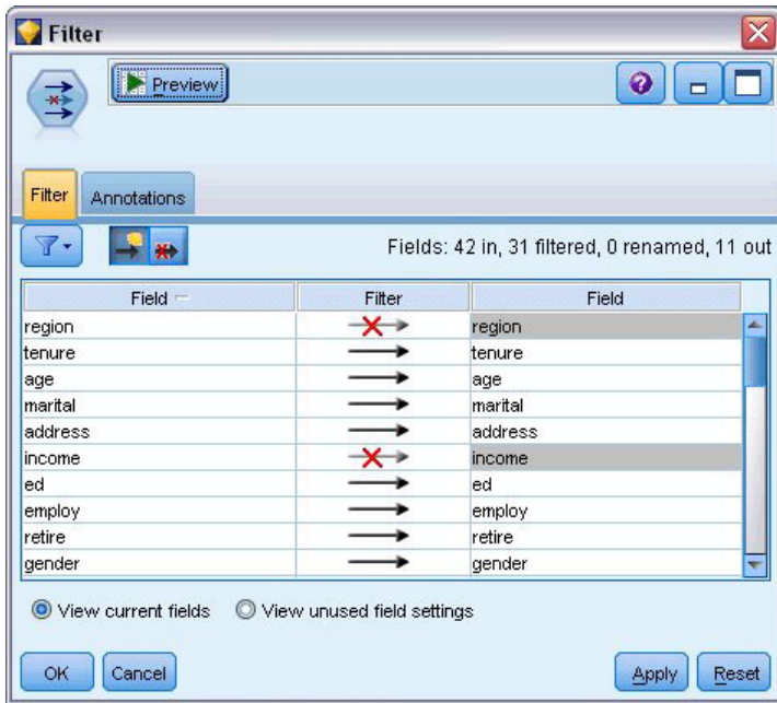
图 245. 过滤不必要的字段
