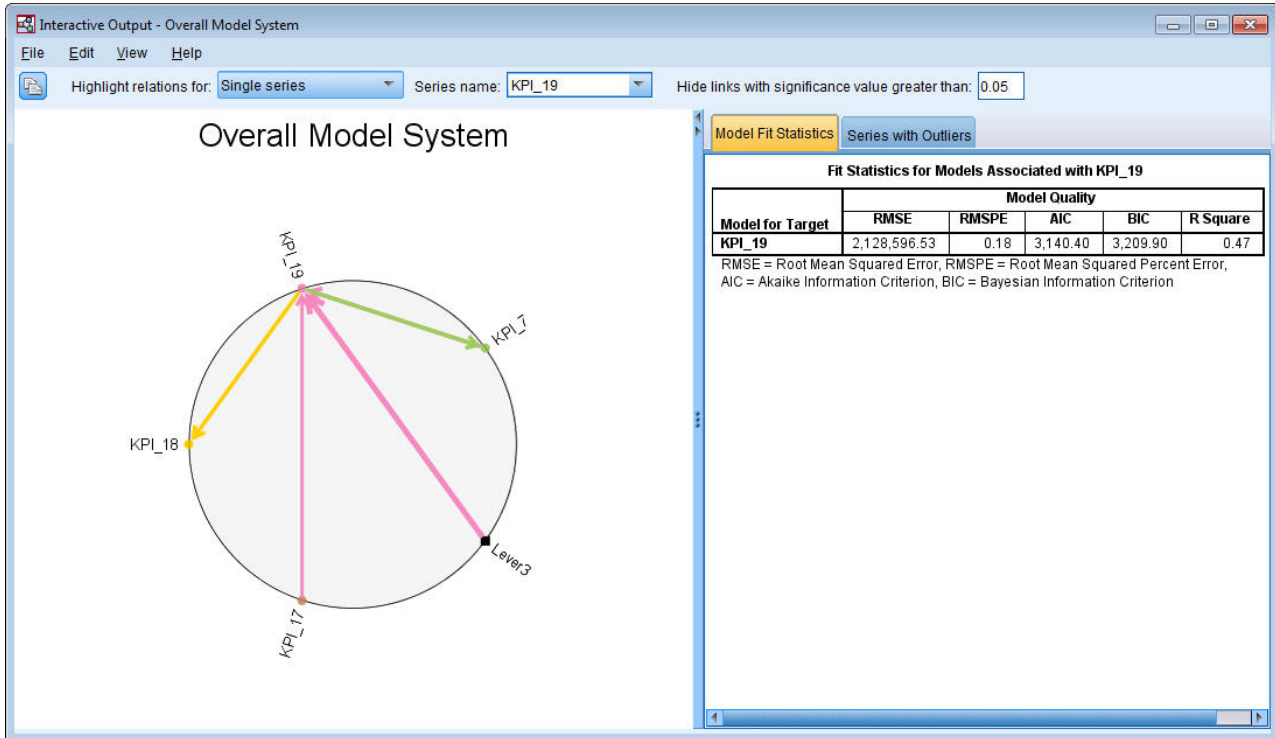
图 406. 总体模型系统，查看单一序列
