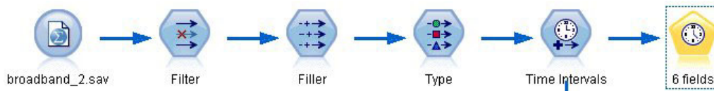
图 196. 将建模节点附加到流
