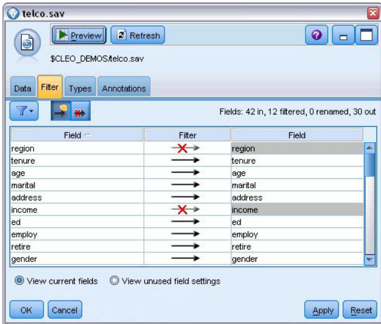
图 344. 过滤不需要的字段
