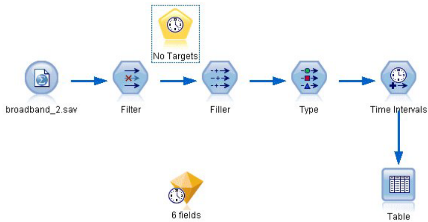
图 195. 从模型块生成建模节点
