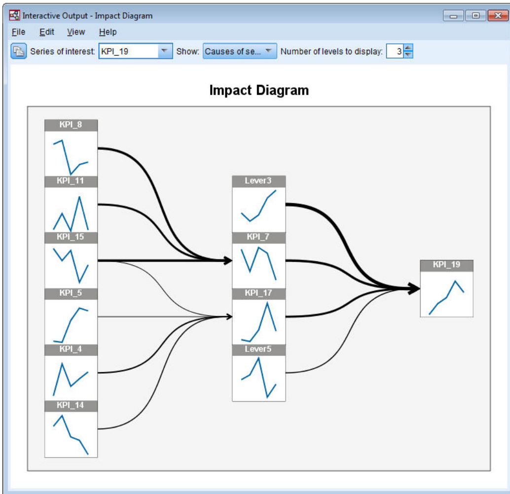
图 409. 因的影响图
