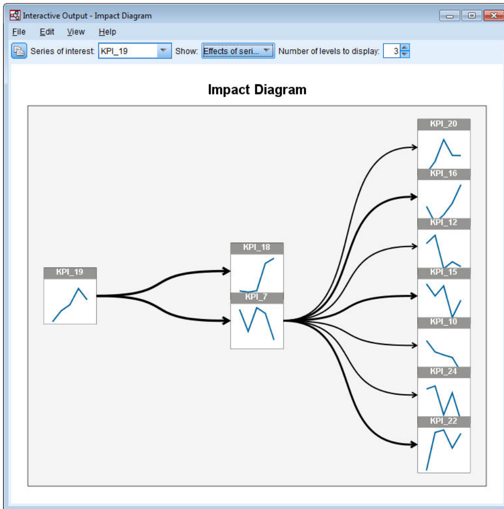
图 408. 效应影响图
