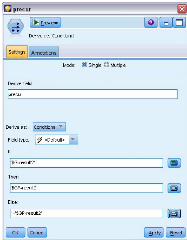
图 312. “派生”节点设置选项
