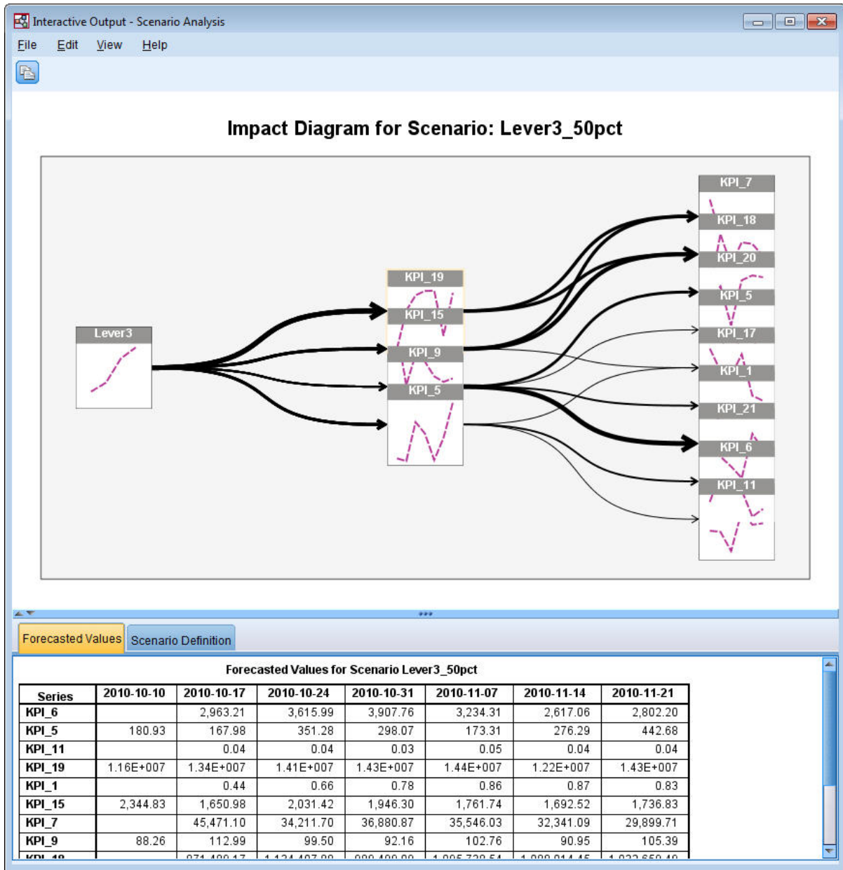
图 416. 方案: Lever3_50pct 的影响图
