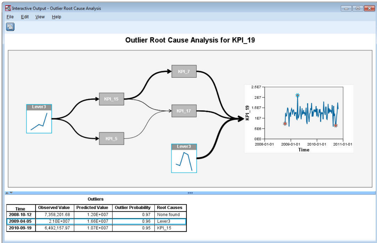
图 412. KPI_19 的离群值根本原因分析
