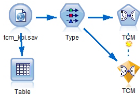
图 401. TCM 建模的样本流
