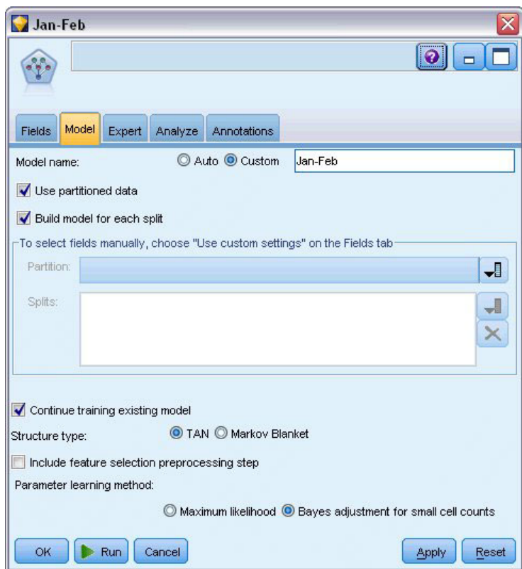
图 249. 重新训练模型
