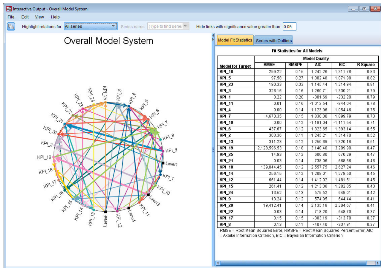
图 405. 总体模型系统，查看所有序列
