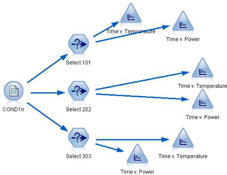
图 263. Condplot 流
