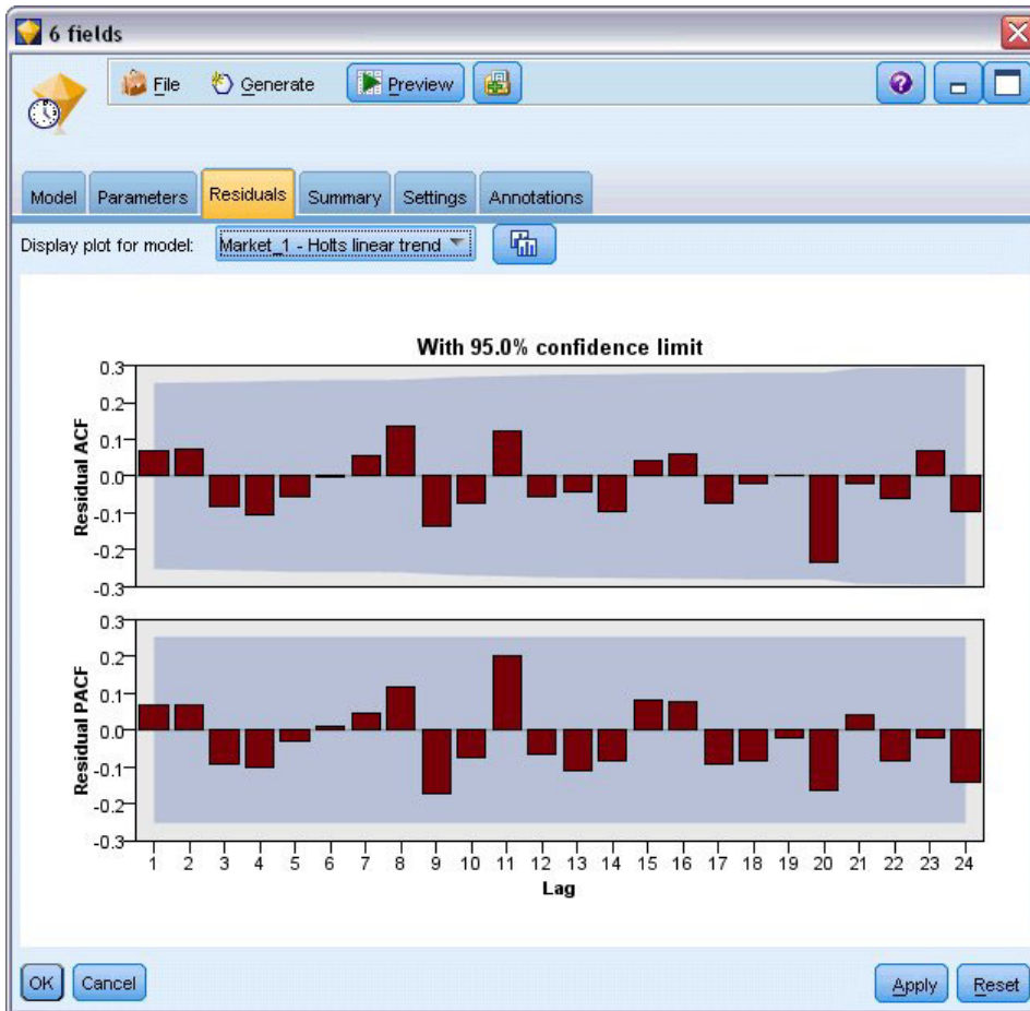
图 186. 市场的 ACF 值和 PACF 值
