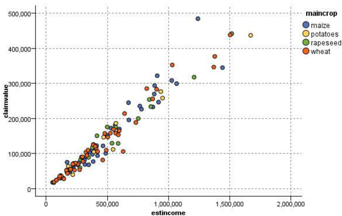
图 28. 将主要作物类型作为交叠来绘制估计收入与索赔值之间关系的散点图
