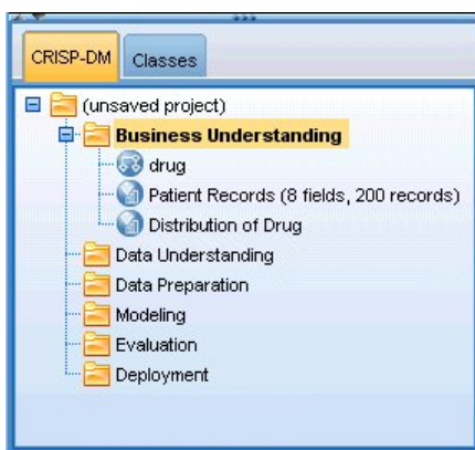
Abbildung 2. CRISP-DM-Projekttool
