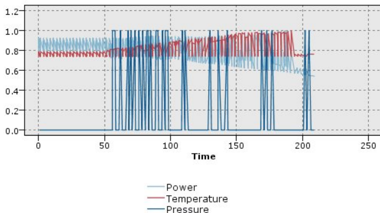
Abbildung 25. Normalisierter Multiplot mit einem Plot für den Druck (Pressure)
