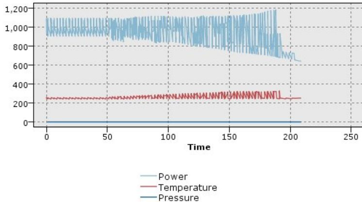
Abbildung 24. Standard-Multiplot mit der Kraftwerksfluktuation im Lauf der Zeit (Hinweis: Ohne Normalisierung ist der Plot für den Druck (Pressure) nicht sichtbar)
