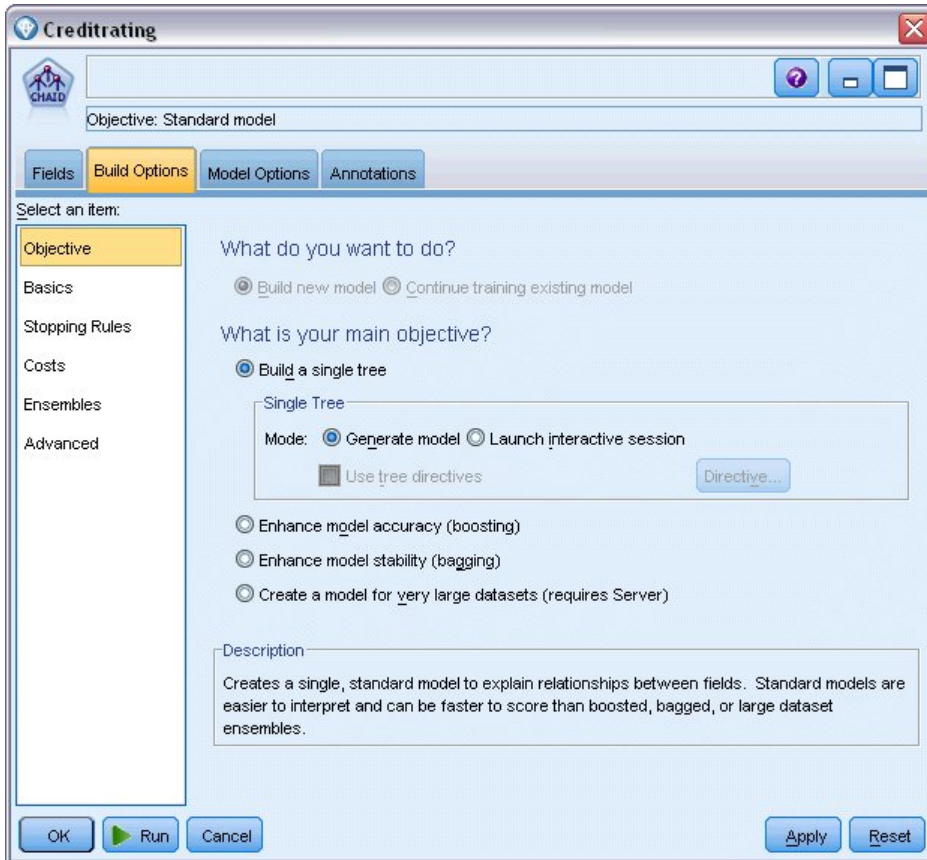
Figura 6. Nodo de modelado CHAID, pestaña Opciones de generación
