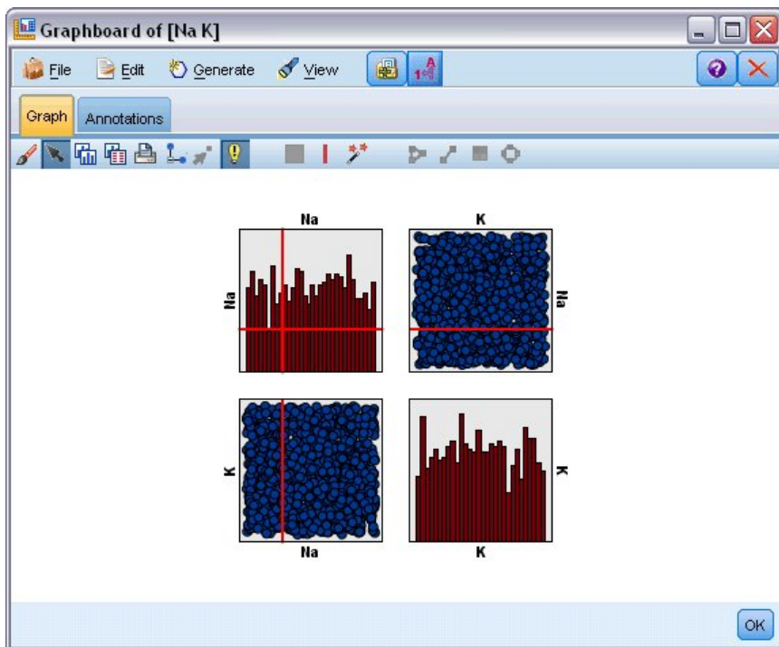
Figura 50. SPLOM con tramos
