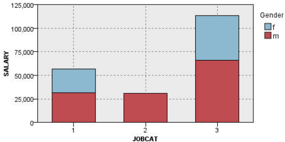
Figura 9. Gráfico de barras apiladas
