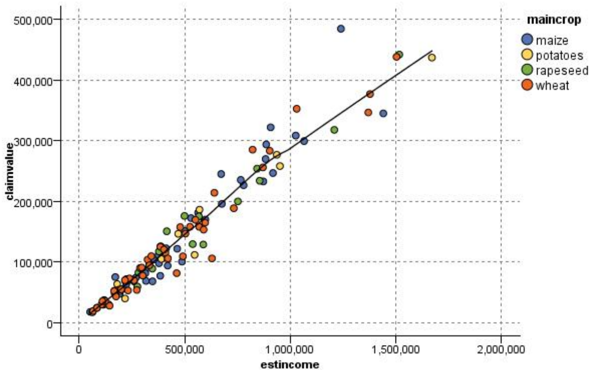
Figura 22. Gráfico con un campo de superposición de suavizamiento LOESS
