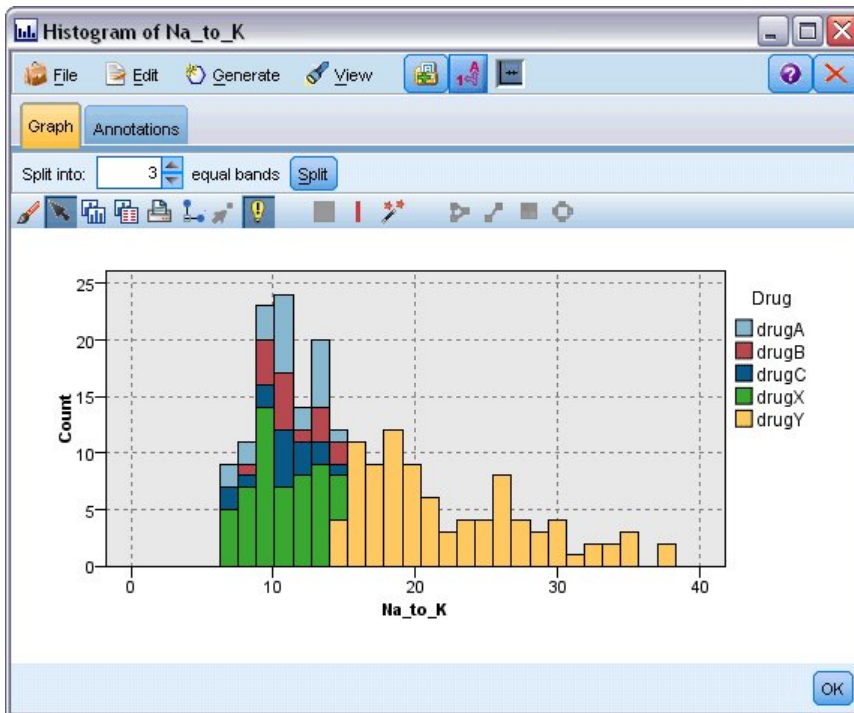
Figura 53. Creación de la barra de herramientas de tramos iguales con tramos activados
