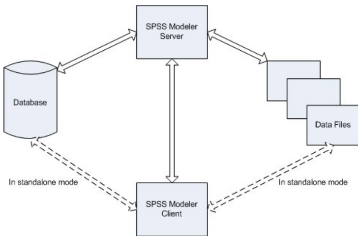
Figura 1. Arquitectura de IBM SPSS Modeler Server
