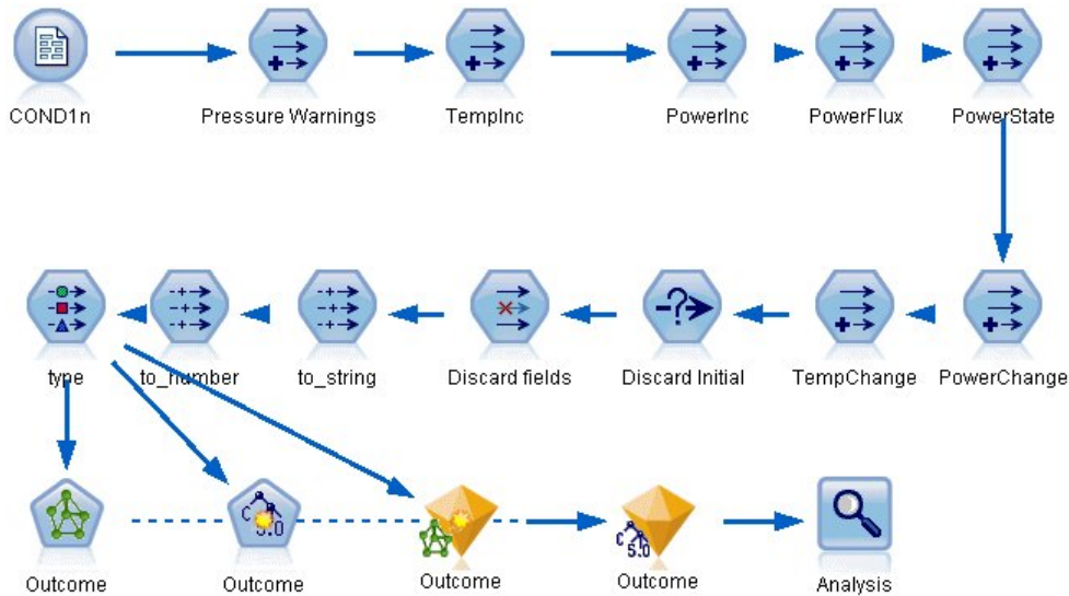
Figure 267. Test du réseau formé
