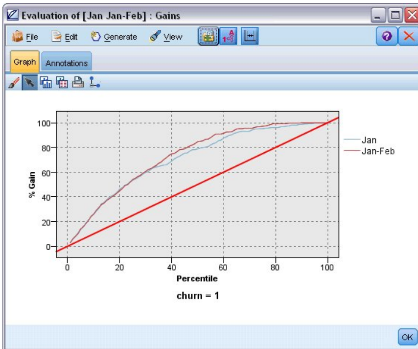
Figure 257. Evaluation de la précision du modèle
