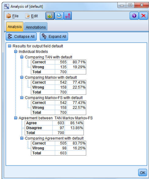
Figure 243. Analyse de la précision des modèles
