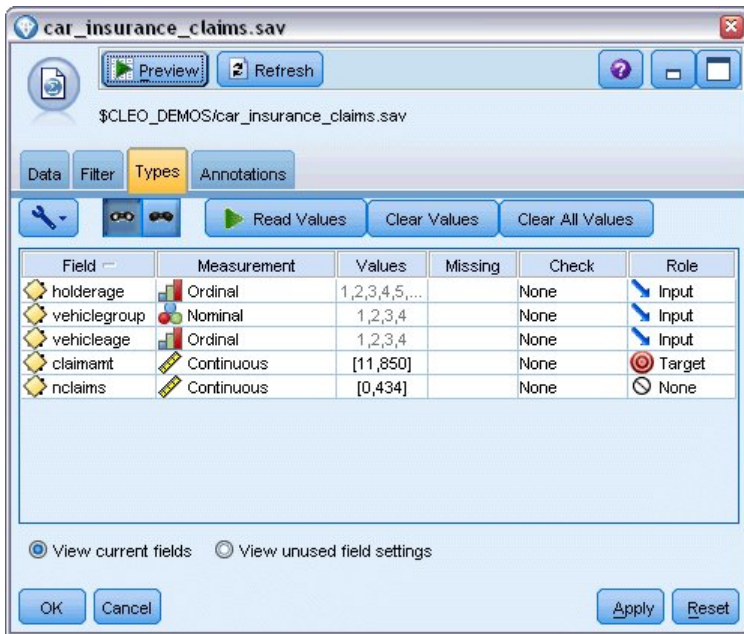
Figure 327. Définition du rôle de champ
