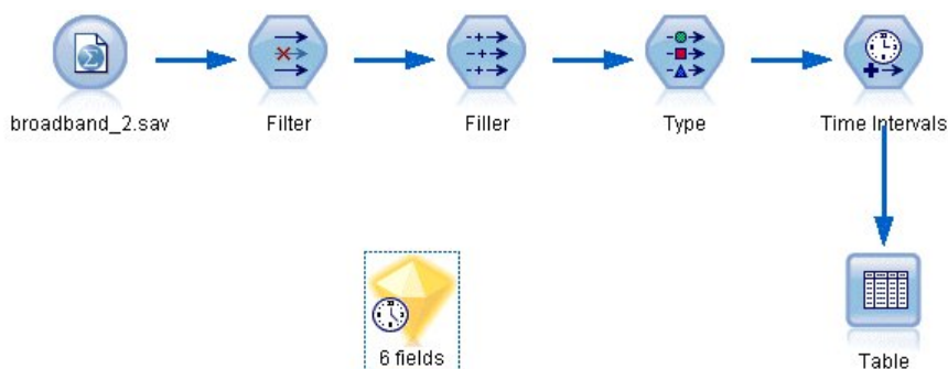
Figure 194. Ajout du nugget de modèle
