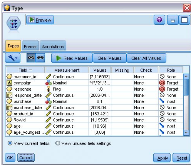
Figure 223. Modification des paramètres du noeud type
