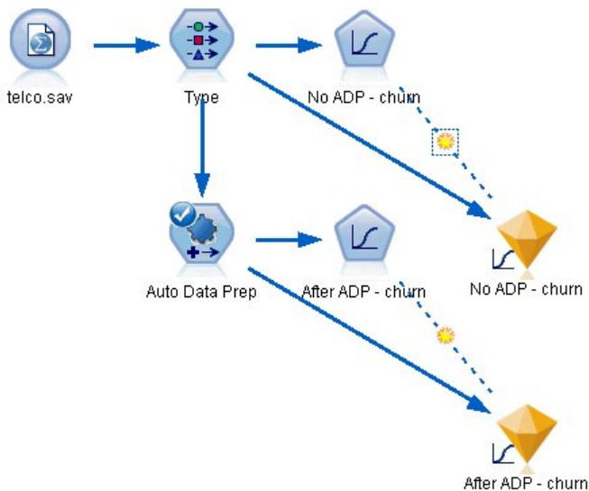
Figure 56. Relier les nuggets de modèle
