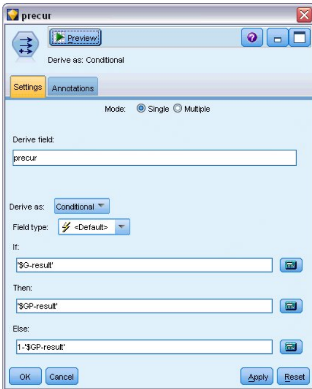
Figure 297. Options des paramètres du noeud Calculer
