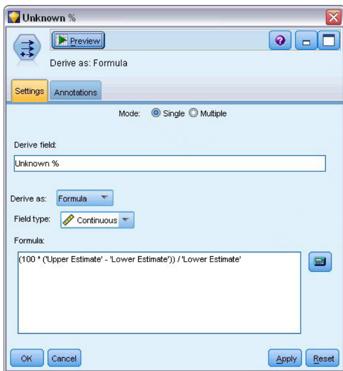
図 373. フィールド作成ノード: 「設定」タブ
