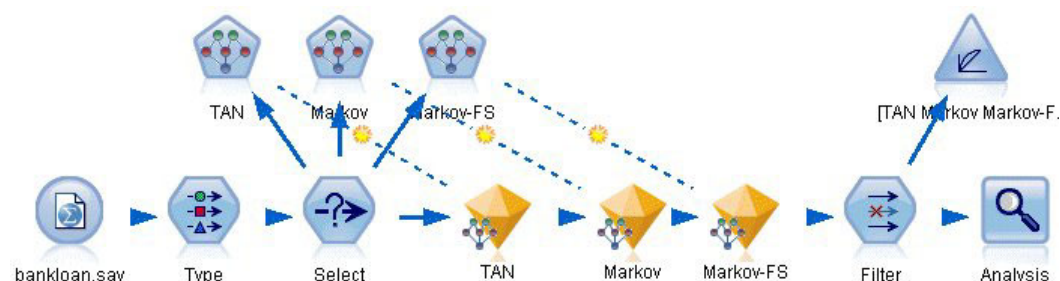
図 233. ベイズ・ネットワークのサンプル・ストリーム
