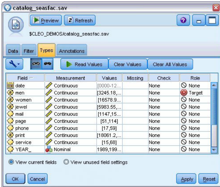
図 202. 対象フィールドの指定
