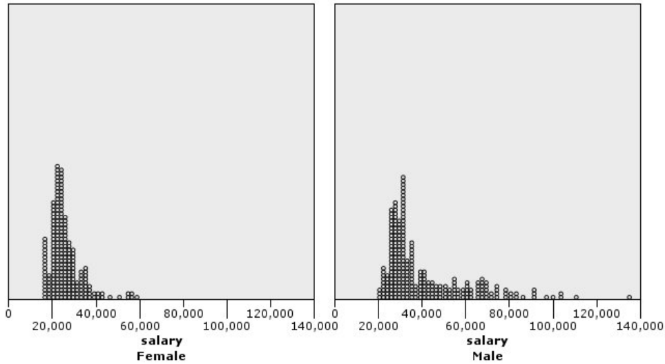
图 11. 点图组
