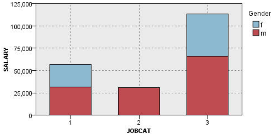
图 9. 堆积条形图
