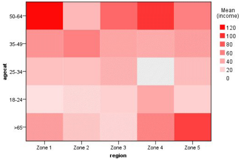
图 14. 分类热图
