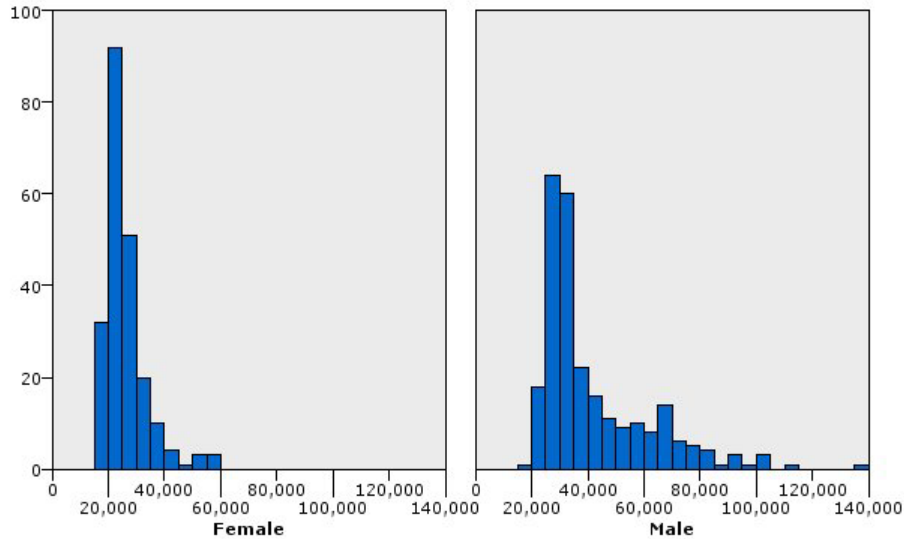
图 10. 直方图组
