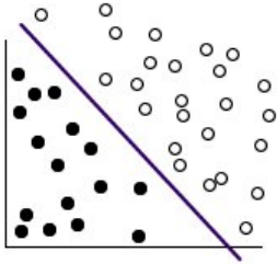
Abbildung 61. Transformierte Daten
