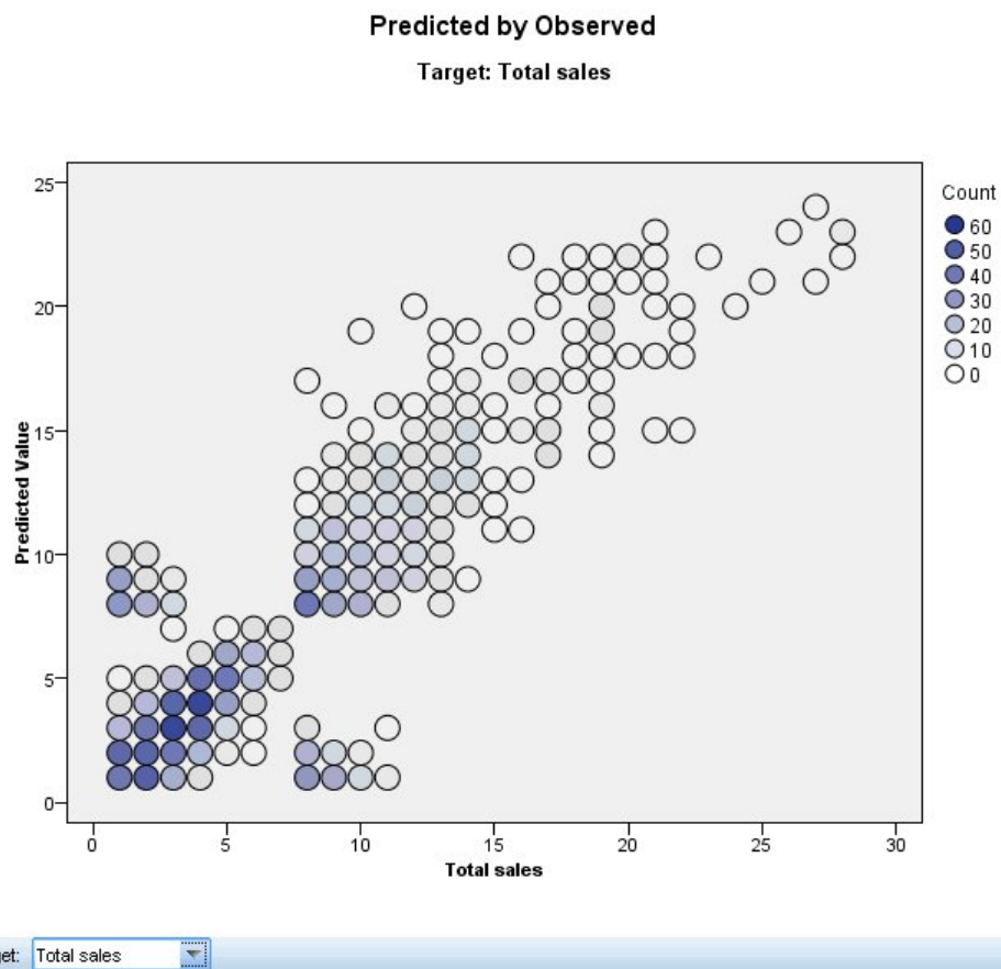
図 40. 「予測対観測」ビュー
