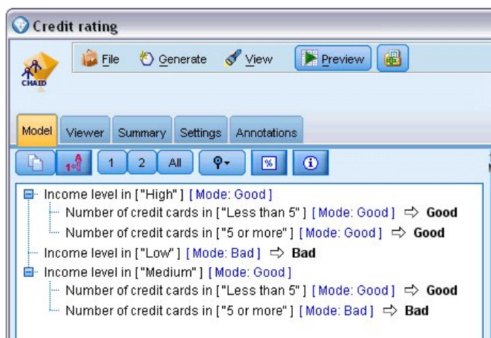
図 9. CHAID モデル・ナゲット、ルール・セット
