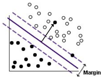
図 64. 線型区分の問題
