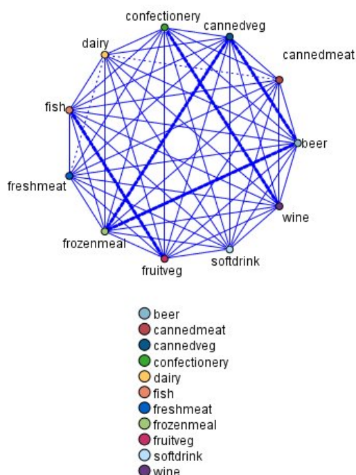
図 45. 買い物かごの品物の関連を示す Web グラフ・ノード
