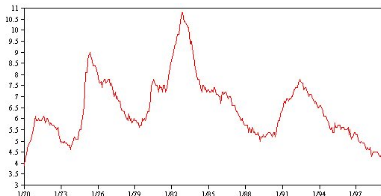
図 55. 非季節性サイクル
