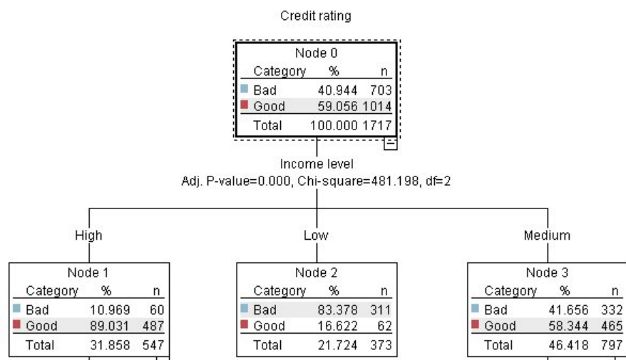
図 1. 簡単なディジジョン・ツリー・モデル
