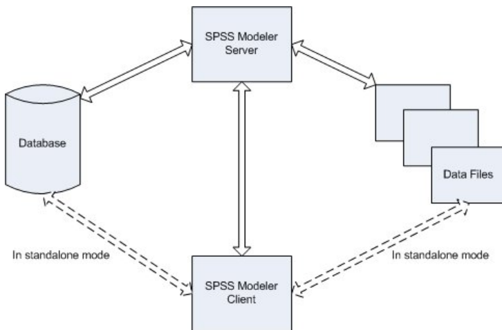
그림 1. IBM SPSS Modeler Server 설계
