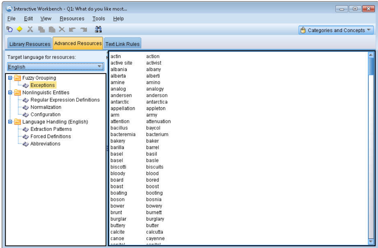
그림 37. 텍스트 마이닝 템플릿 편집기 - 고급 자원 탭
