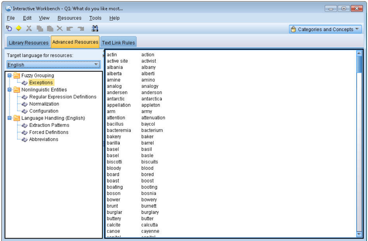
그림 40. 텍스트 마이닝 템플릿 편집기 - 고급 자원 탭
