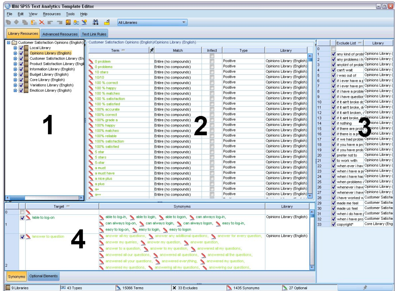
그림 36. 텍스트 마이닝 템플릿 편집기
