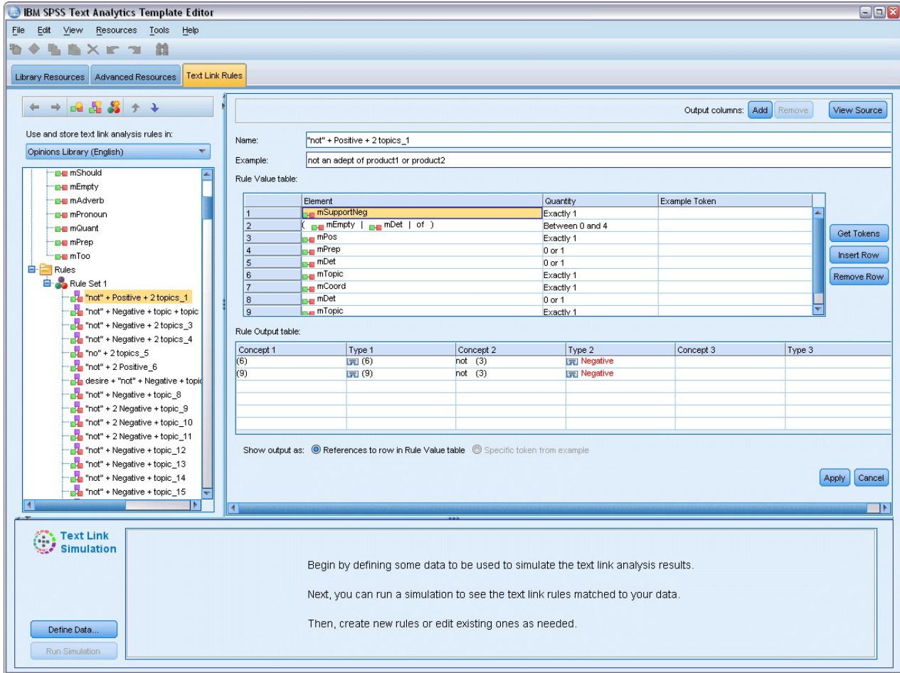
그림 41. 텍스트 링크 규칙 탭
