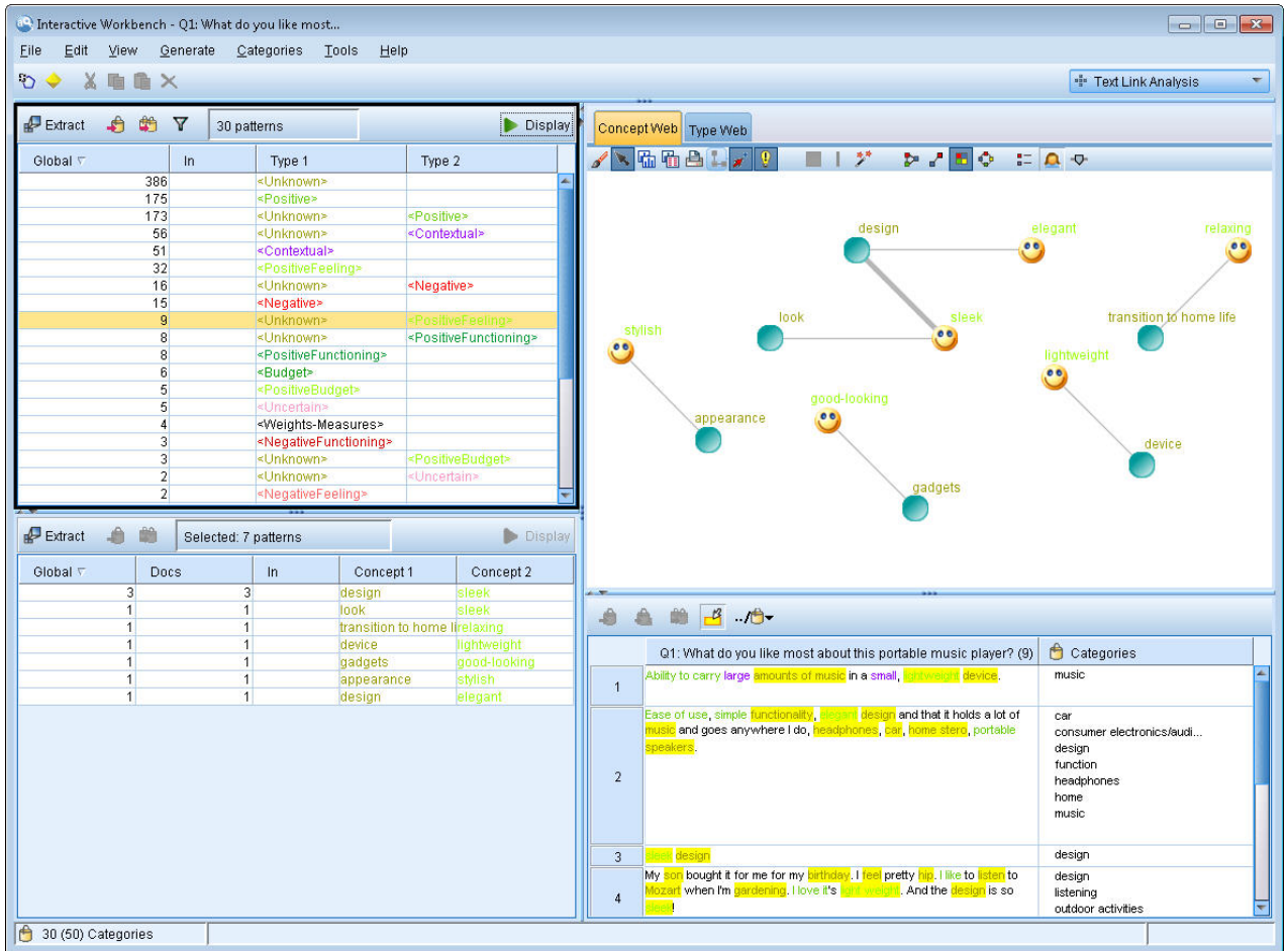
그림 32. 텍스트 링크 분석 보기
