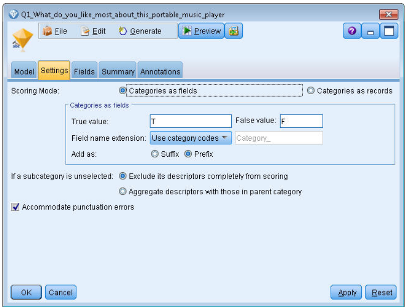
그림 12. 범주 모델 너깃 대화 상자: 설정 탭
