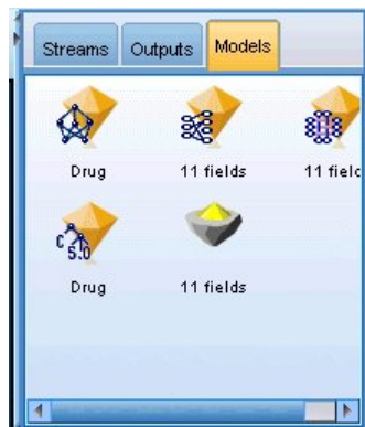
Рисунок 26. Палитра моделей
