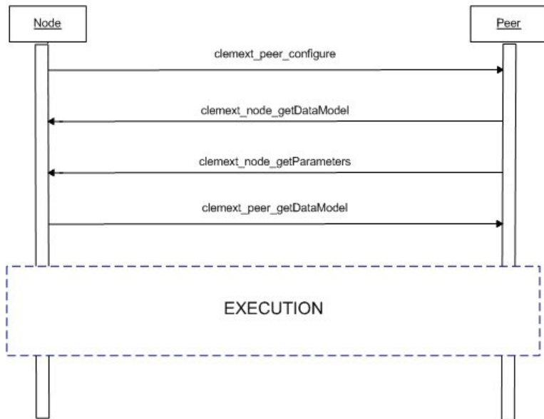
图 97. 典型对等/节点交互块
