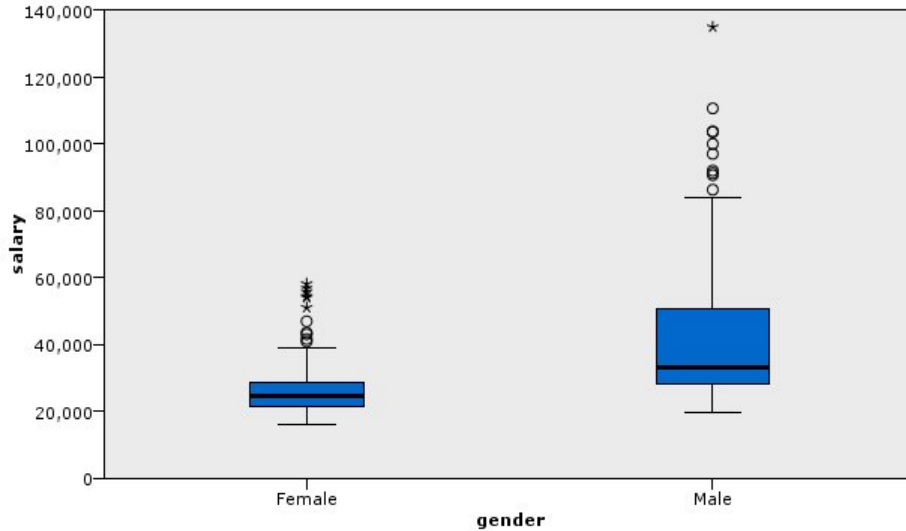
图 12. 箱图
