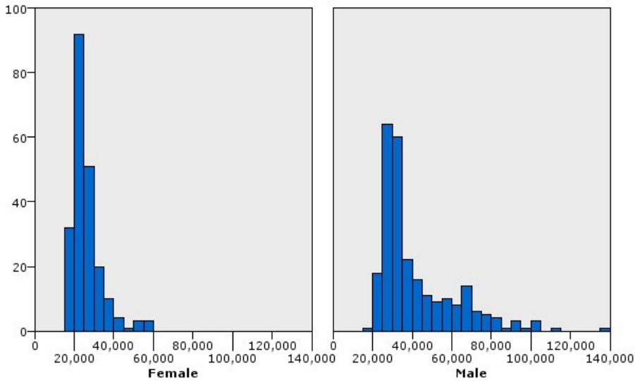
图 10. 直方图组
