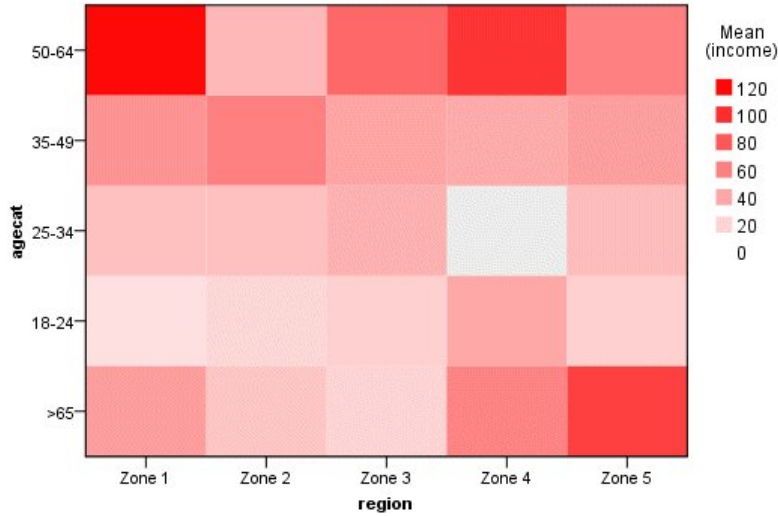
图 14. 分类热图
