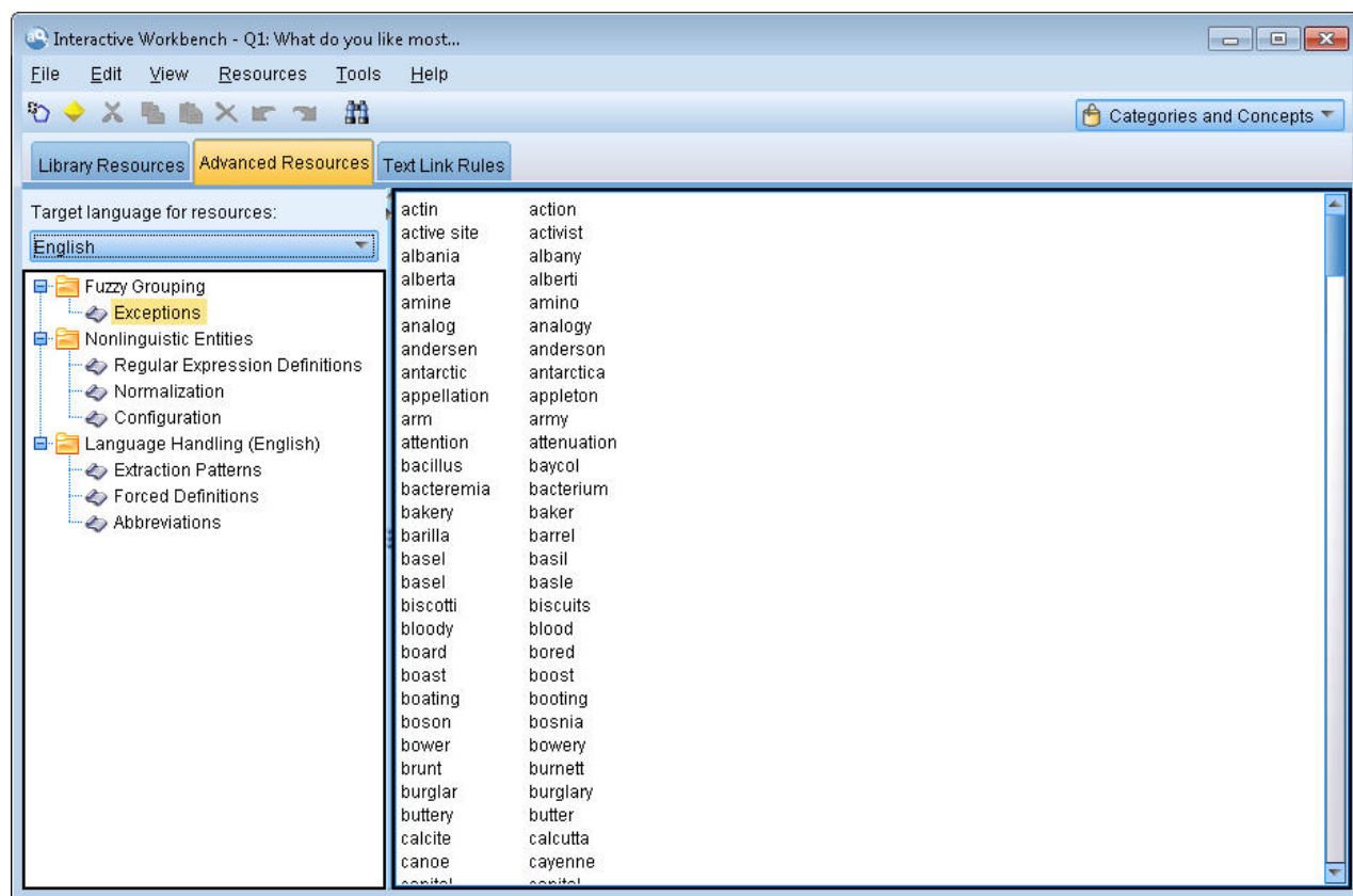
圖 40. 文字挖掘範本編輯器 - 進階資源標籤
