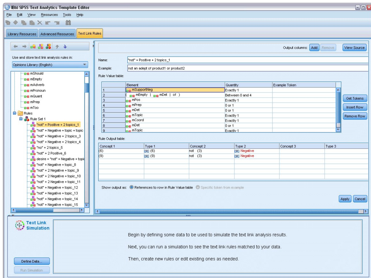
圖 38. 文字採礦範本編輯器 - 文字鏈結規則標籤
