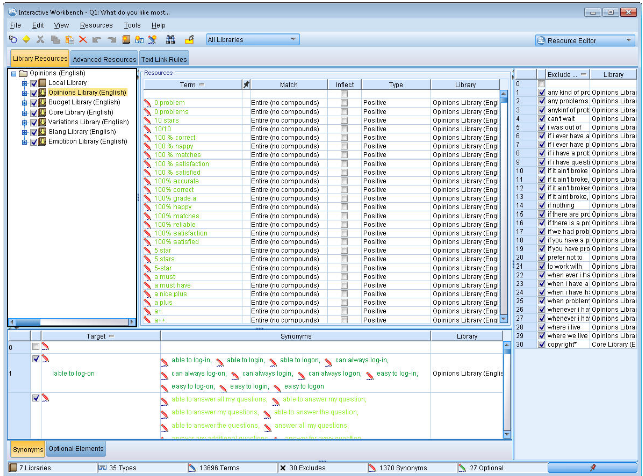
圖 35. 資源編輯器視圖
