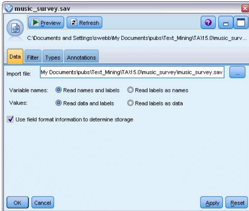
圖 16. 「統計資料檔案」節點對話框：「資料」標籤
