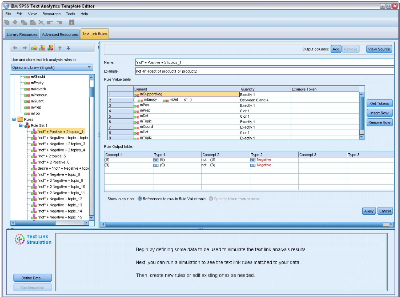
圖 41. 「文字鏈結規則」標籤
