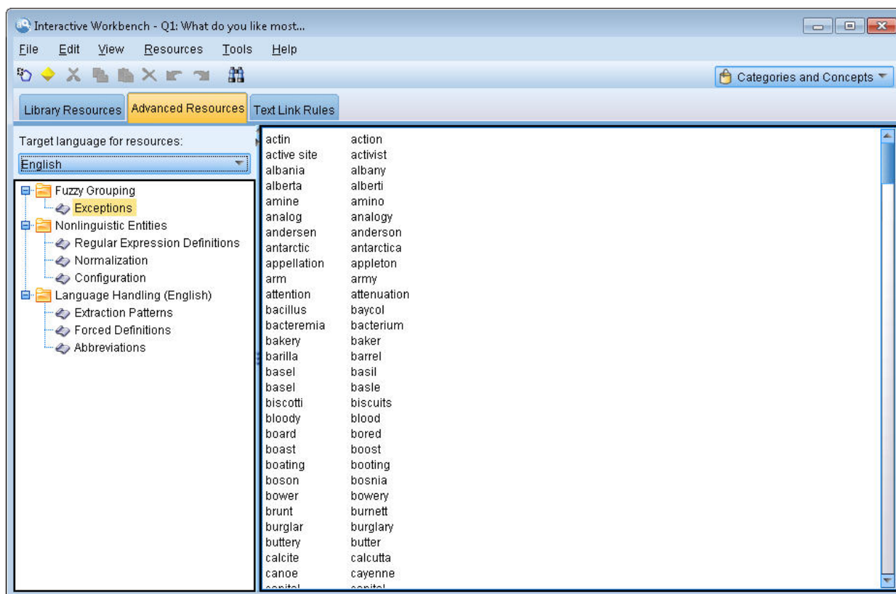
圖 37. 文字挖掘範本編輯器 - 進階資源標籤
