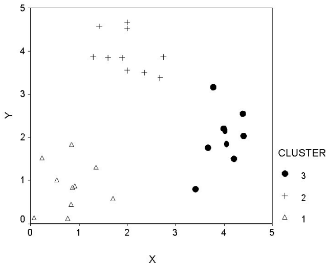
Abbildung 44. Einfaches Clustering-Modell
