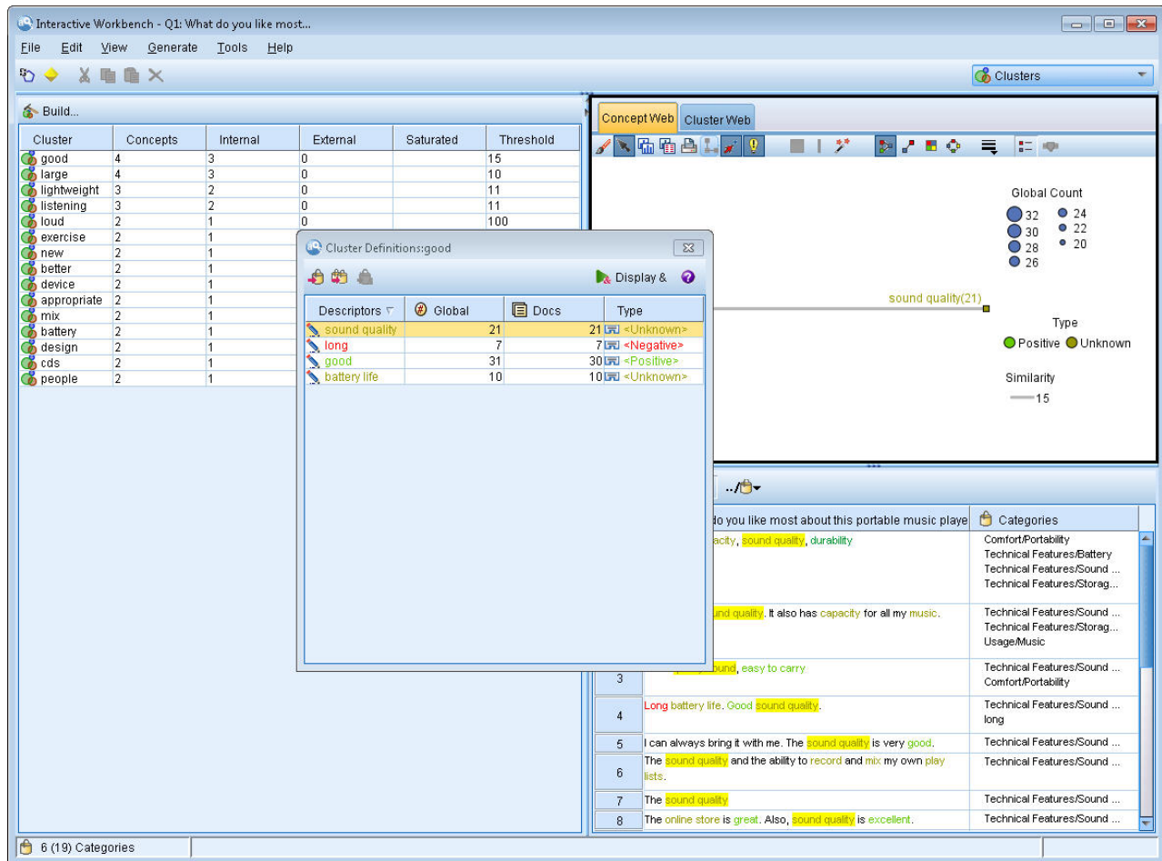
Figure 24. Vue Clusters
