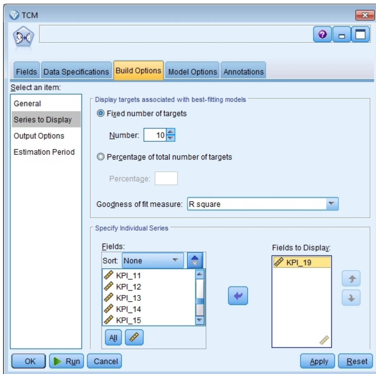
図 407. 時間的因果モデルの表示する系列
