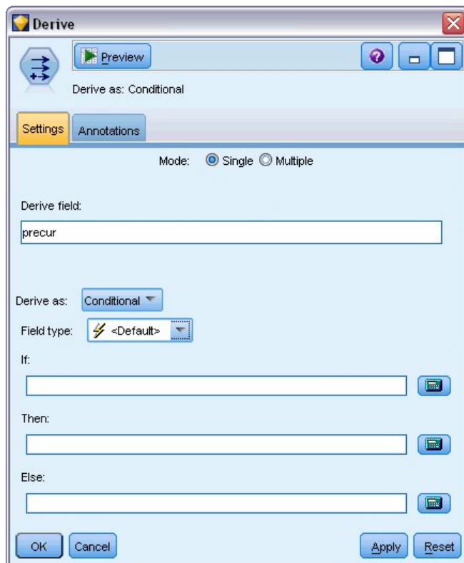
図 305. フィールド作成ノードの設定オプション
