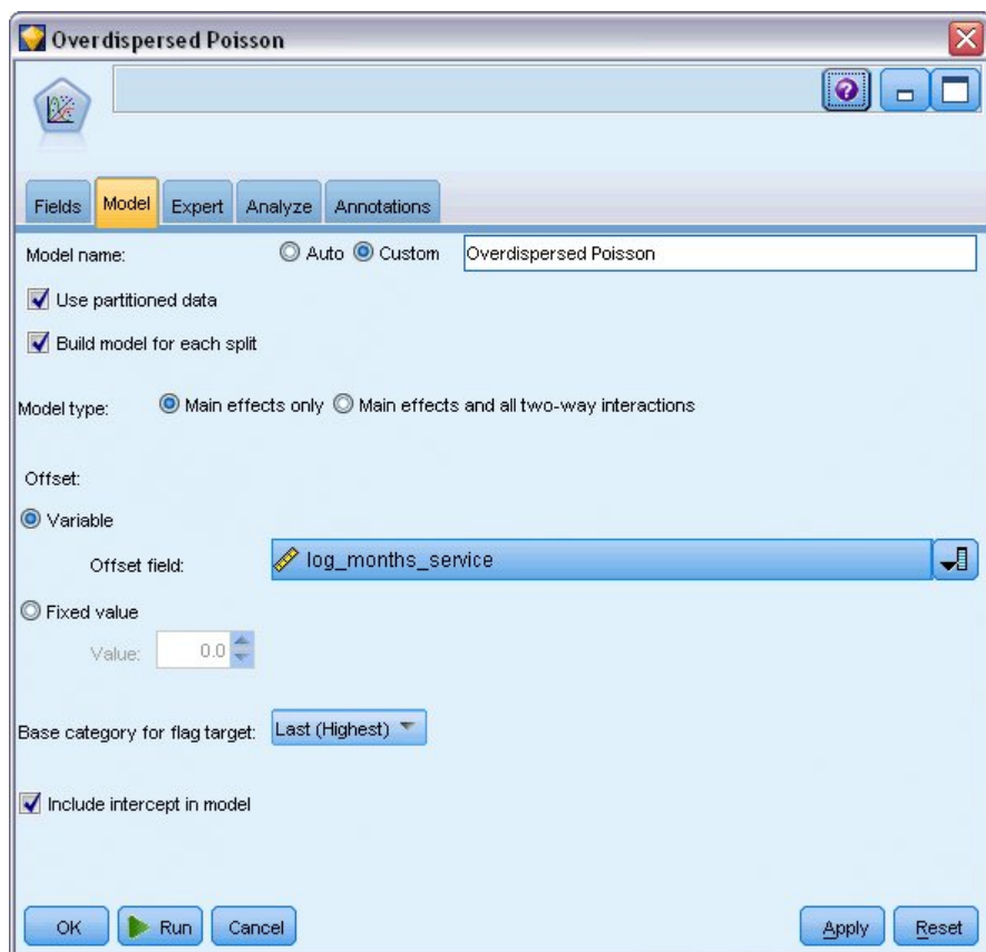
図 314. モデル・オプションの選択
