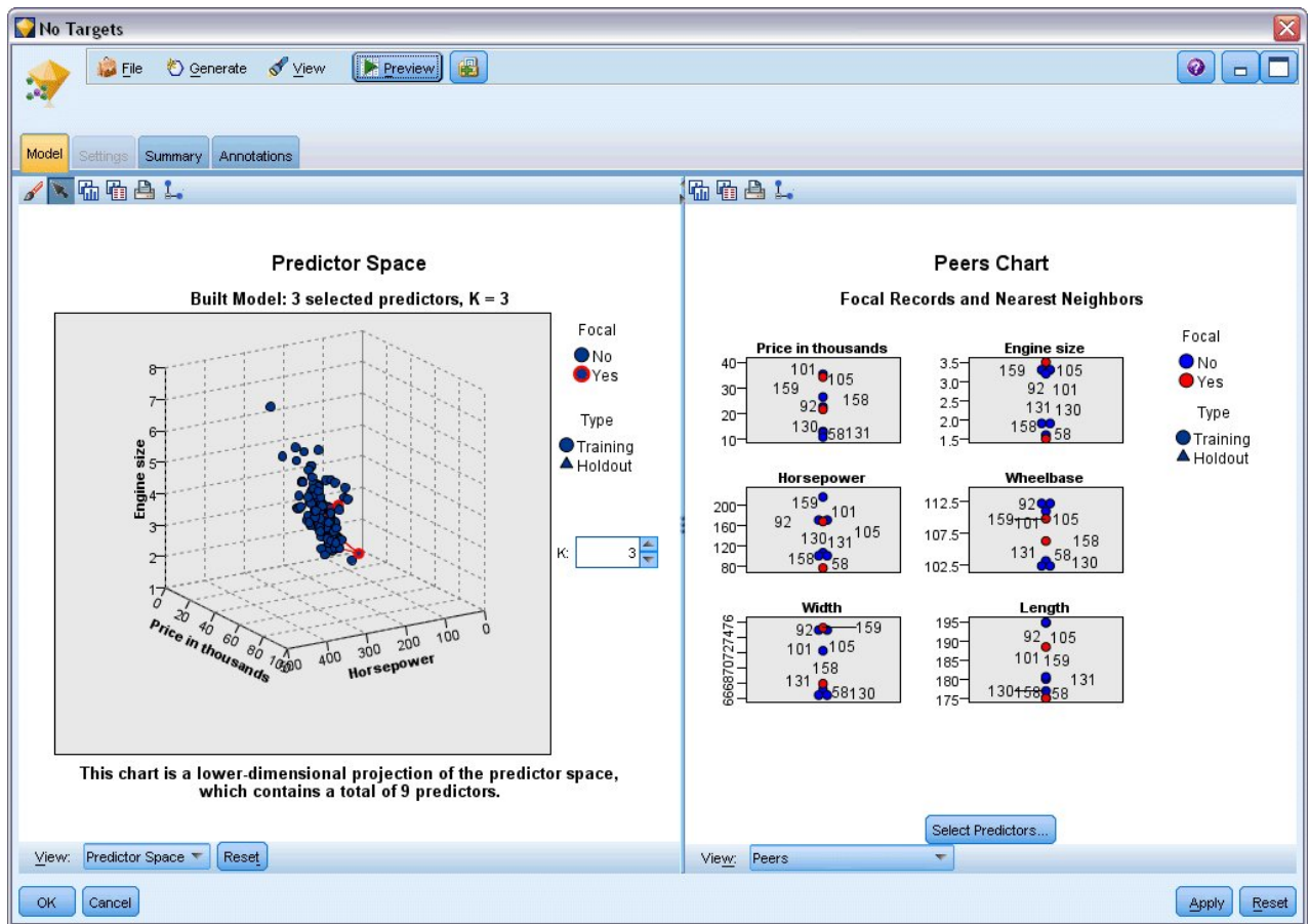
図 392. モデル・ビューアー・ウィンドウ
