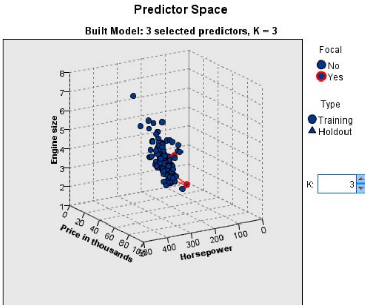
図 393. 予測領域のグラフ
