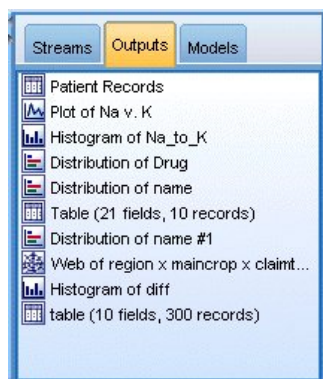
図 6. 「出力」タブ
