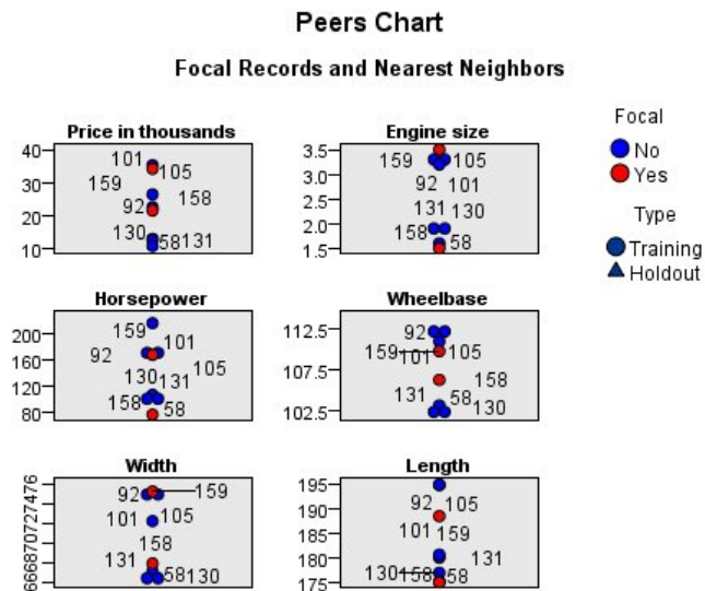
図 396. 同位図の特徴の比較
