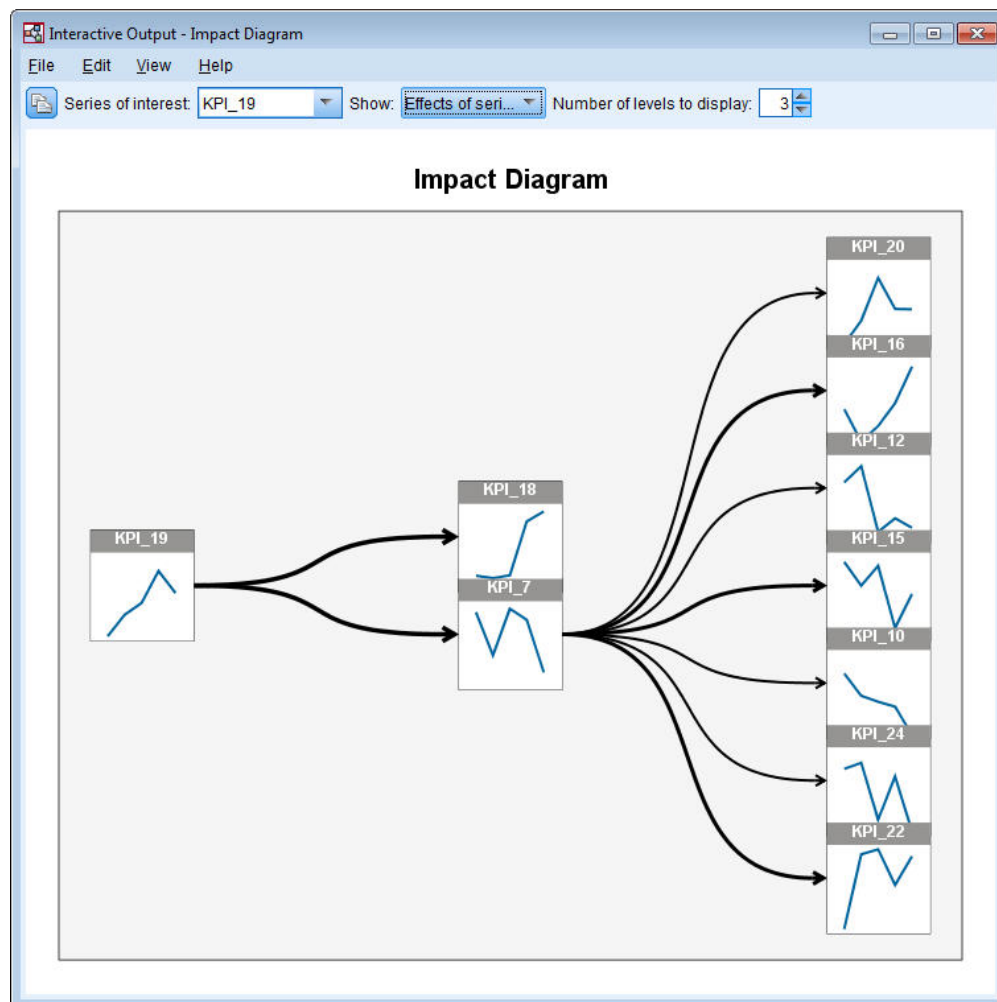
図 405. 効果の影響図
