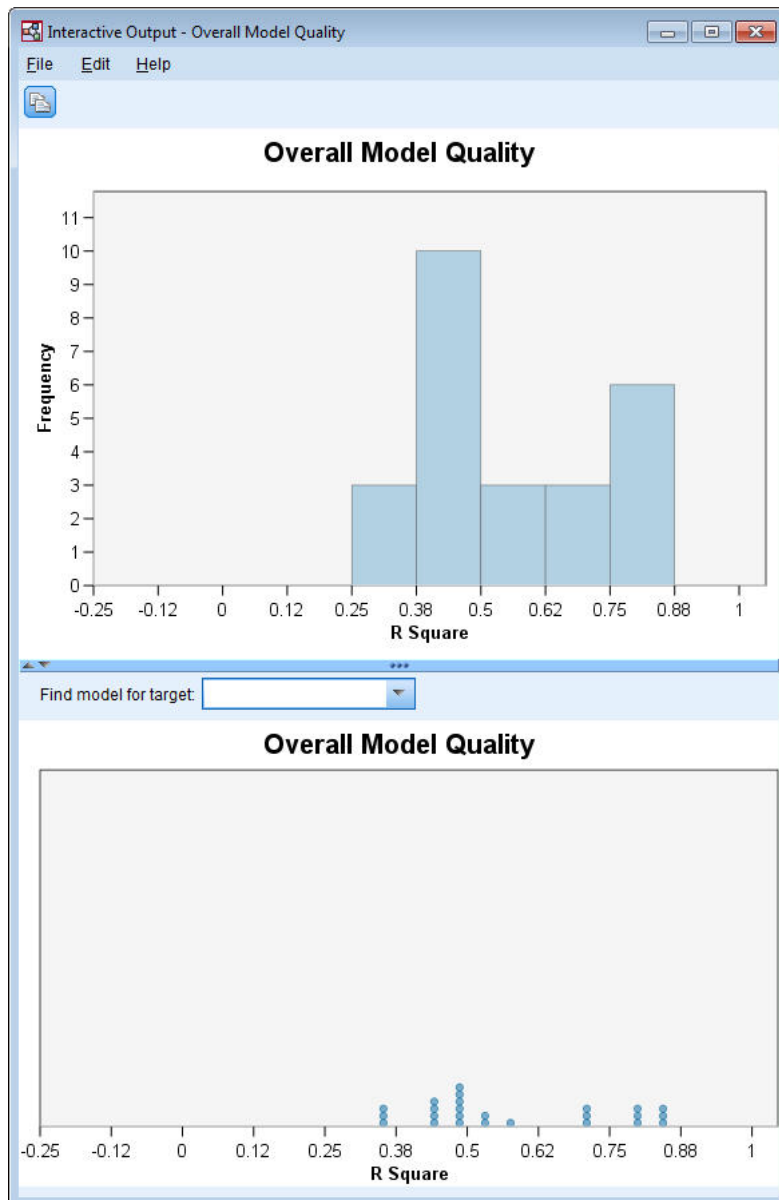
図 401. 全体のモデル品質
