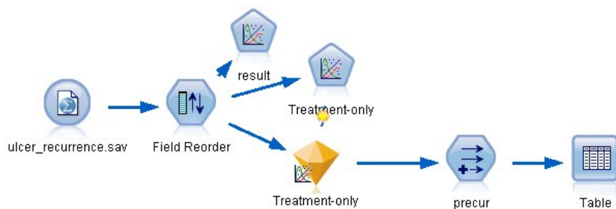
図 281. 潰瘍の再発を予測するサンプル・ストリーム
