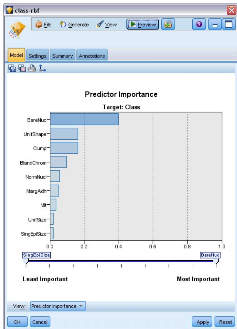
図 334. 予測重要度グラフ
