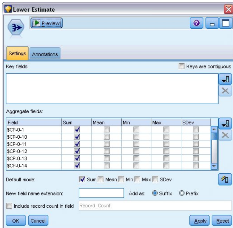
図 361. 集計ノード: 「設定」タブ
