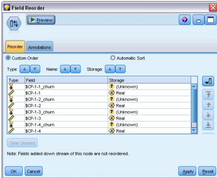
図 378. フィールドの並べ替えノード: 「並べ替え」タブ
