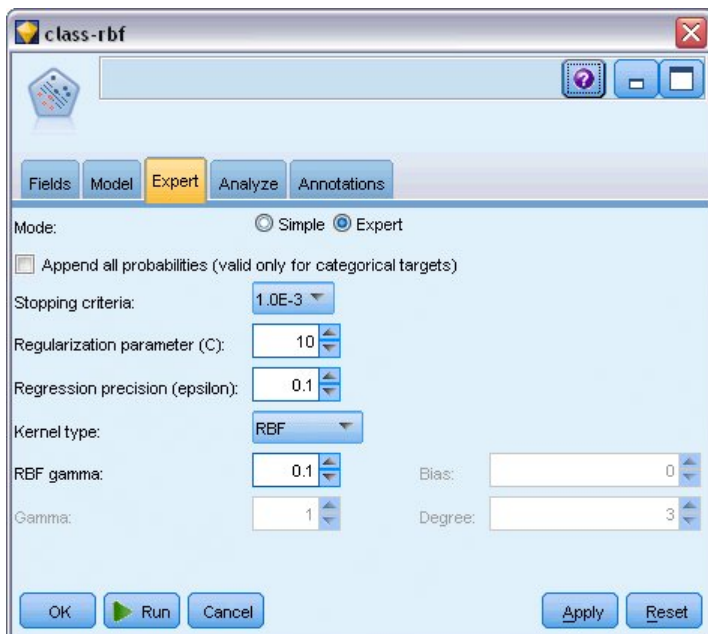
図 332. デフォルトの「エキスパート」タブの設定
