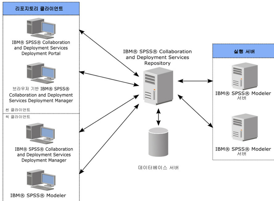
그림 1. IBM SPSS Collaboration and Deployment Services 아키텍처
