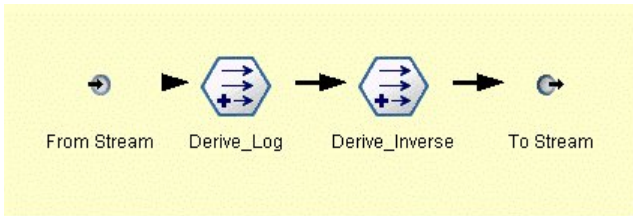
그림 64. 캔버스의 수퍼노드
