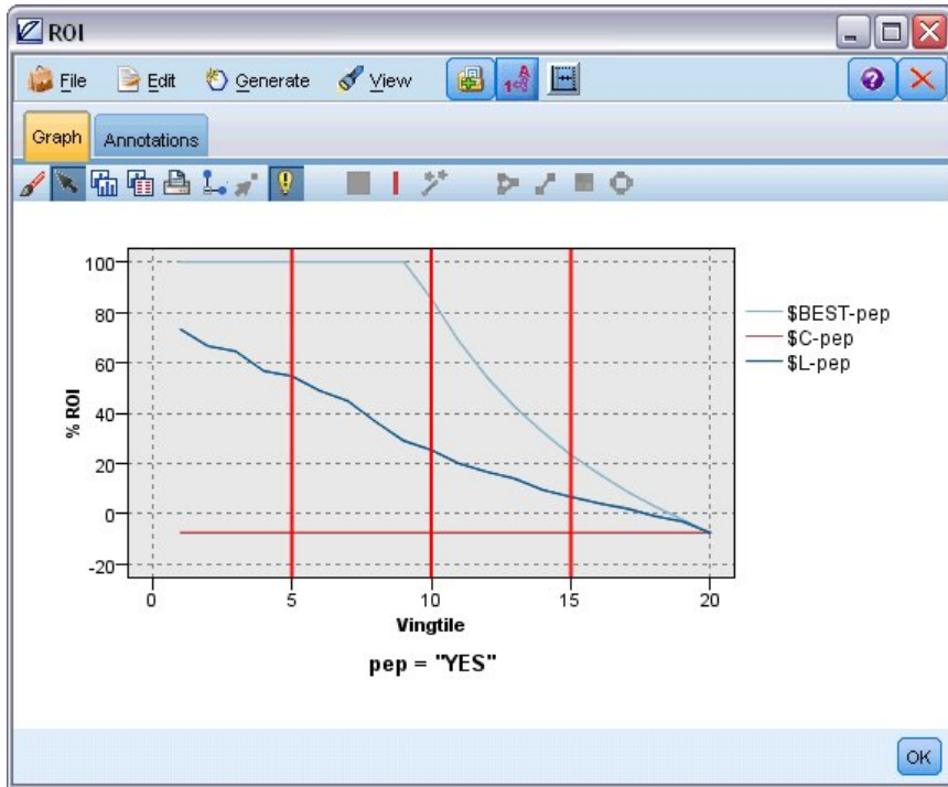
그림 49. 3개의 밴드가 있는 그래프
