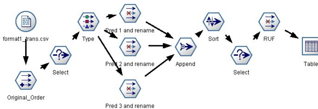
Rysunek 51. Przykładowy strumień służący do transponowania danych transakcyjnych do formatu kasowego
