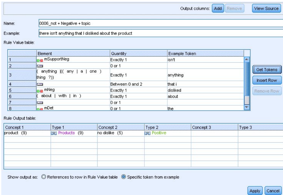
Рисунок 43. Вкладка правил TLA: редактор правил
