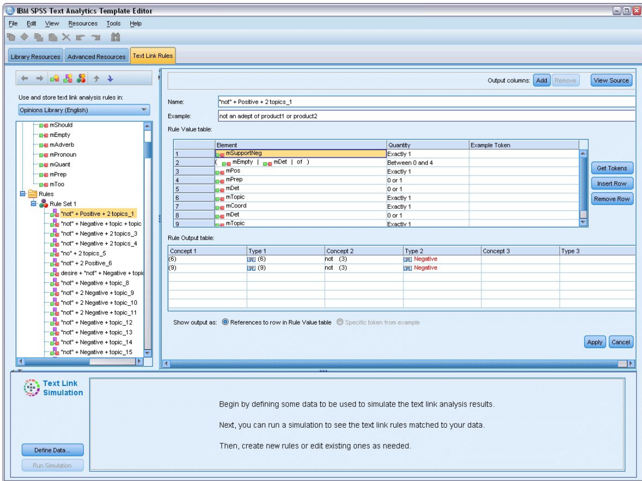
Рисунок 42. Вкладка Правила текстовых связей
