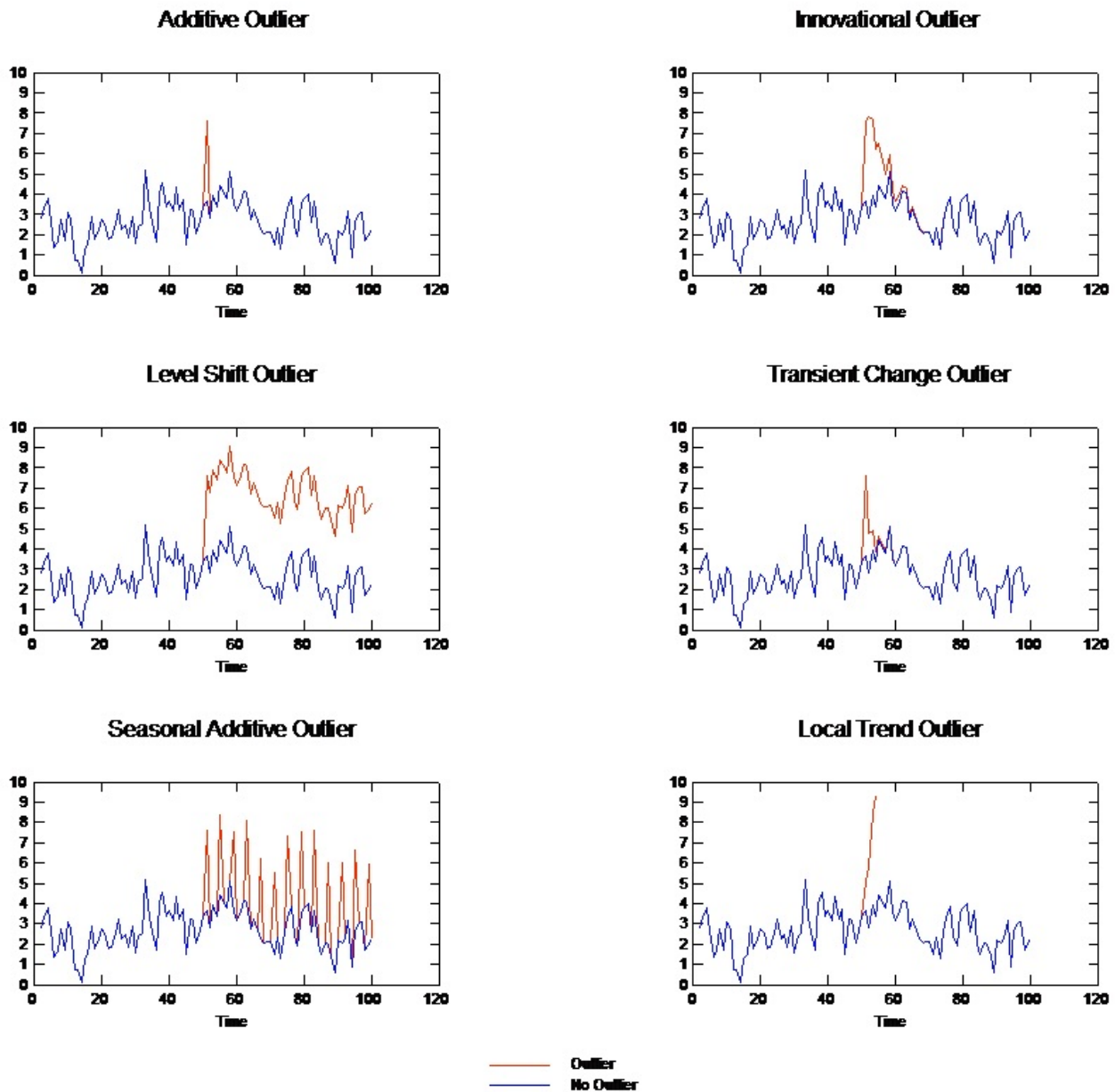
图 57. 离群值类型
