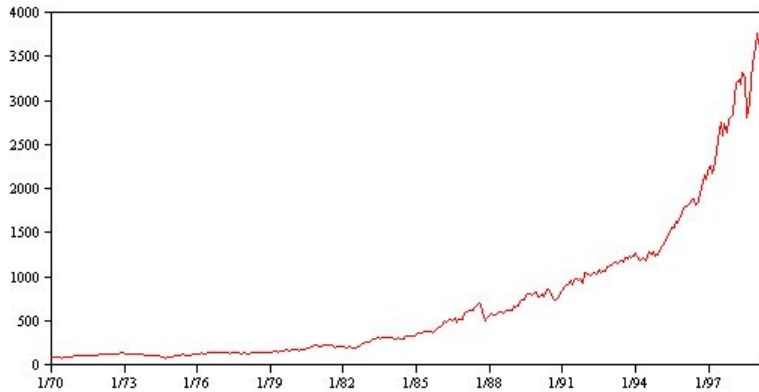
图 53. 趋势
