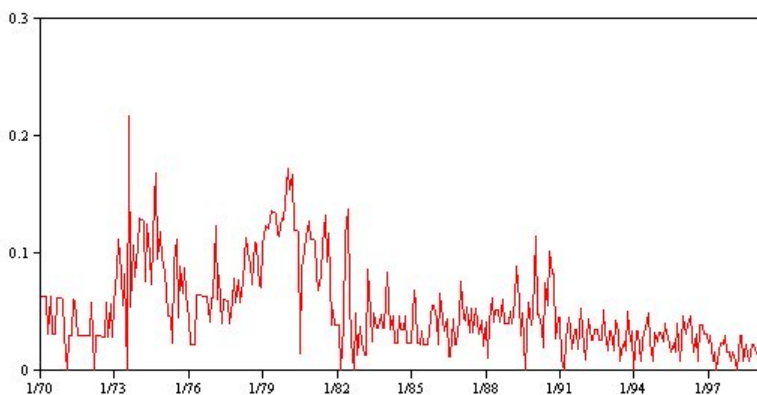
图 56. 脉冲序列
