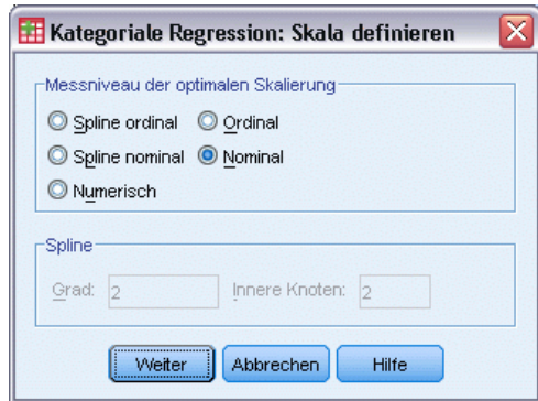
Abbildung 9-11 Dialogfeld “Skala definieren”
