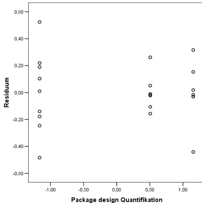
Abbildung 9-24 Residuen bei der kategorialen Regression
