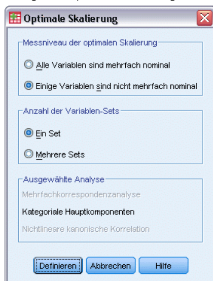
Abbildung 3-1 Dialogfeld "Optimale Skalierung"
