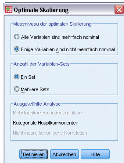
Abbildung 10-1 Dialogfeld "Optimale Skalierung"
