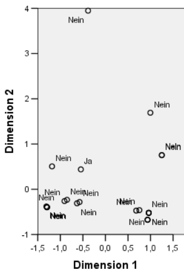
Abbildung 13-12 Objektwerte beschriftet mit "Messing"
