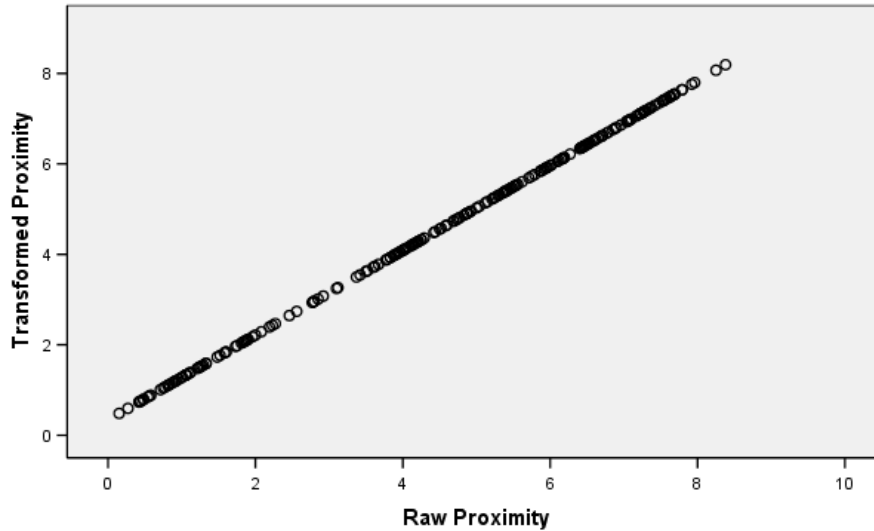
Abbildung 15-30 Transformationsdiagramm
