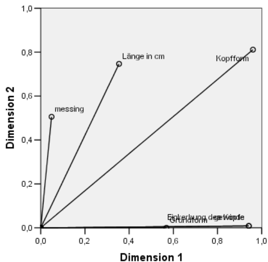
Abbildung 13-16 Diskriminationsmaße
