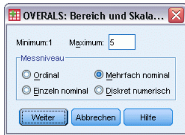
Abbildung 11-6 Dialogfeld "Bereich und Skala definieren"
