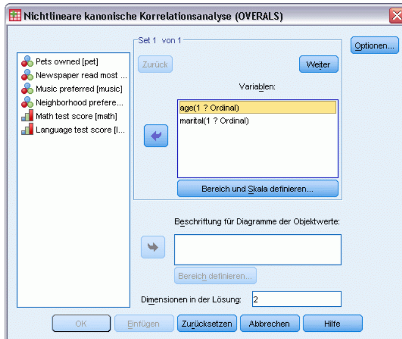
Abbildung 4-2 Dialogfeld "Nichtlineare kanonische Korrelationsanalyse (OVERALS)"
