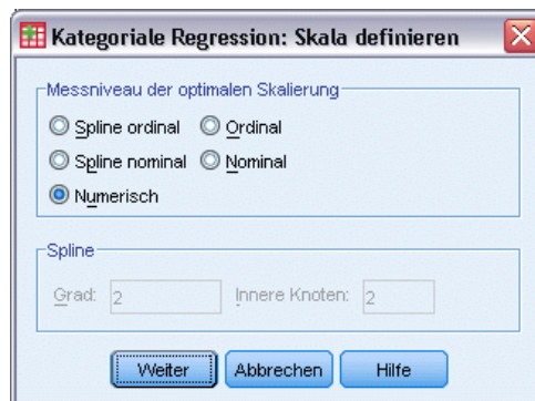
Abbildung 9-26 Dialogfeld "Skala definieren"
