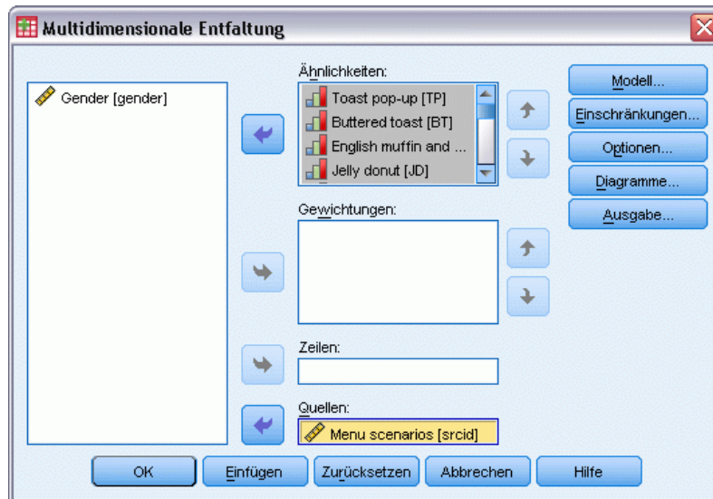
Abbildung 8-1 Hauptdialogfeld "Multidimensionale Entfaltung"
