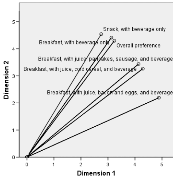
Abbildung 15-15 Dimensionsgewichtungen
