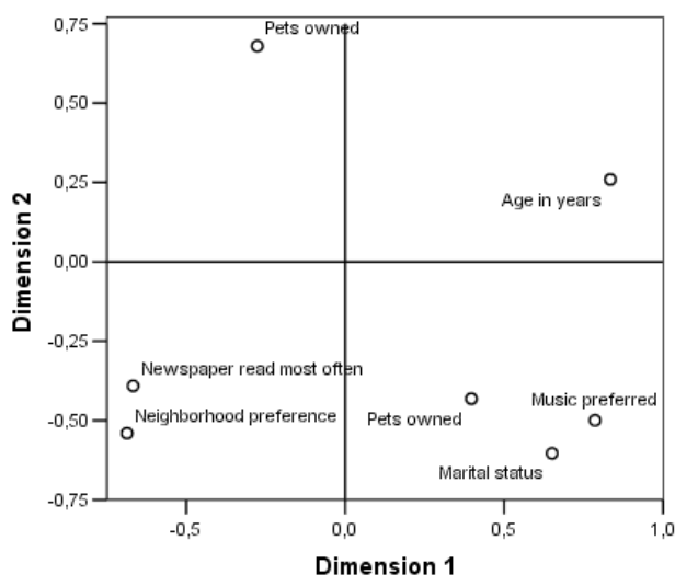
Abbildung 11-17 Komponentenladungen
