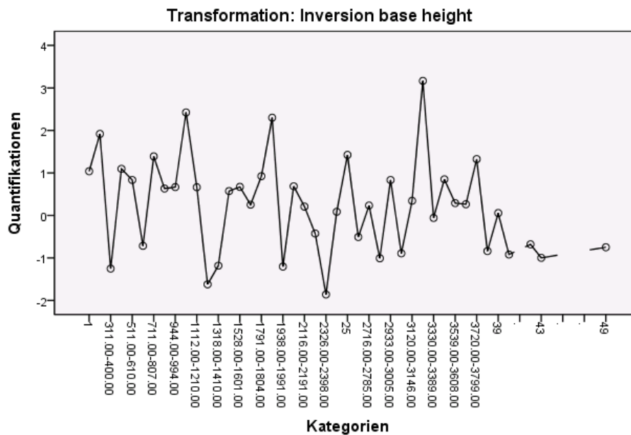
Abbildung 9-32 Transformationsdiagramm von "Inversion base height" (nominal)
