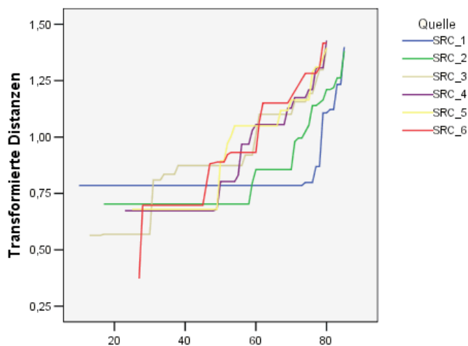
Abbildung 14-18 Transformierte Ähnlichkeiten
