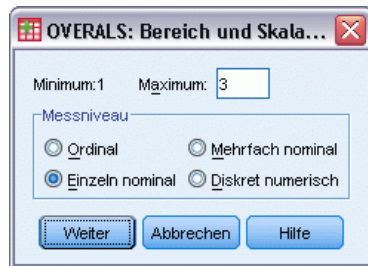
Abbildung 11-10 Dialogfeld "Bereich und Skala definieren"
