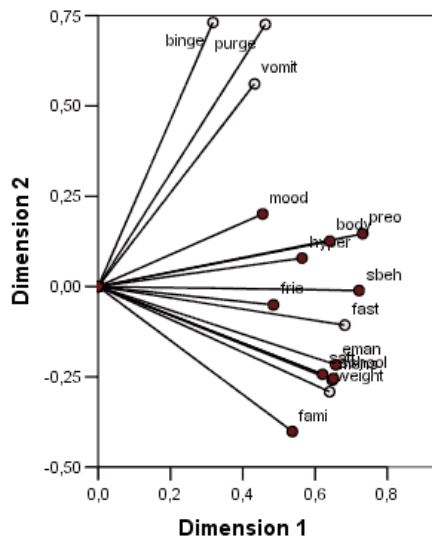
Abbildung 10-36 Komponentenladungsdiagramme
