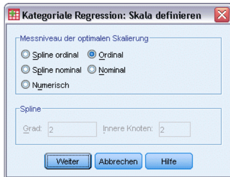
Abbildung 9-37 Dialogfeld “Skala definieren”
