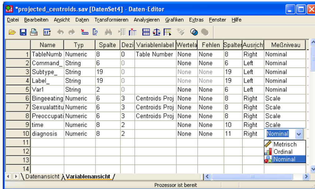
Abbildung 10-48 Projected_centroids.sav
