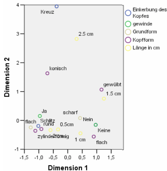
Abbildung 13-8 Kategorienquantifikationen
