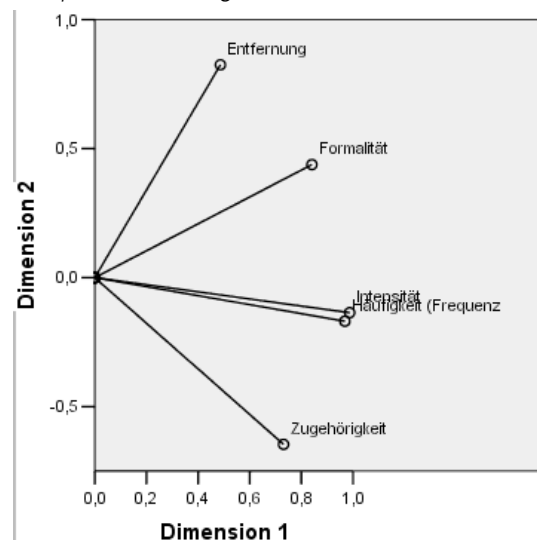
Abbildung 10-13 Komponentenladungen
